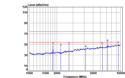
Sub_TX_CH_L_Horizontal
