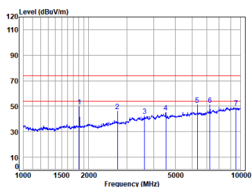
Sub_TX_CH_L_Vertical
