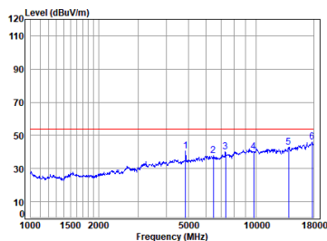
11b_TX_CH_06_Vertical-Avg
