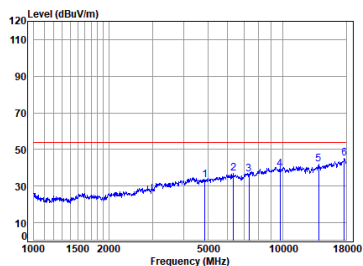
11g_TX_CH_06_Vertical-Avg
