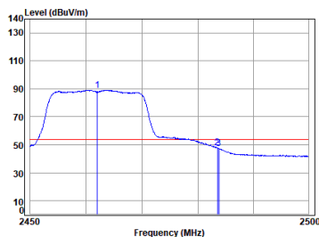
11g_TX_CH_11_Vertical-Avg
