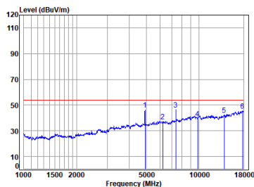
11b_TX_CH_11_Vertical-Avg
