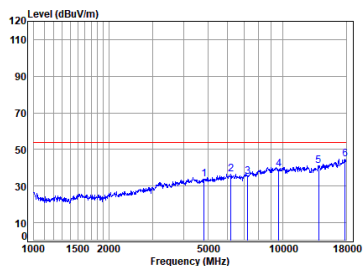
11g_TX_CH_01_Vertical-Avg
