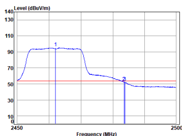
11g_TX_CH_11_Horizontal-Avg
