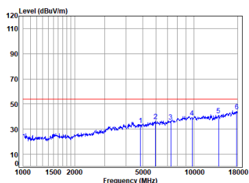
11g_TX_CH_06_Horizontal-Avg
