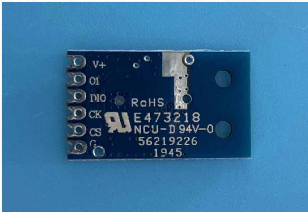
EUT Photo
