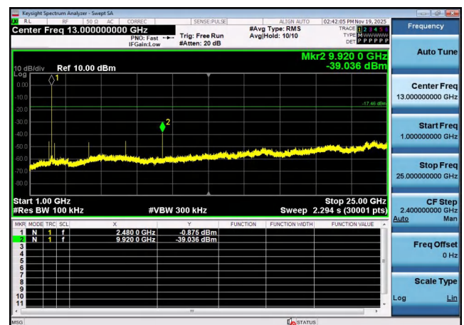
1G-25G
