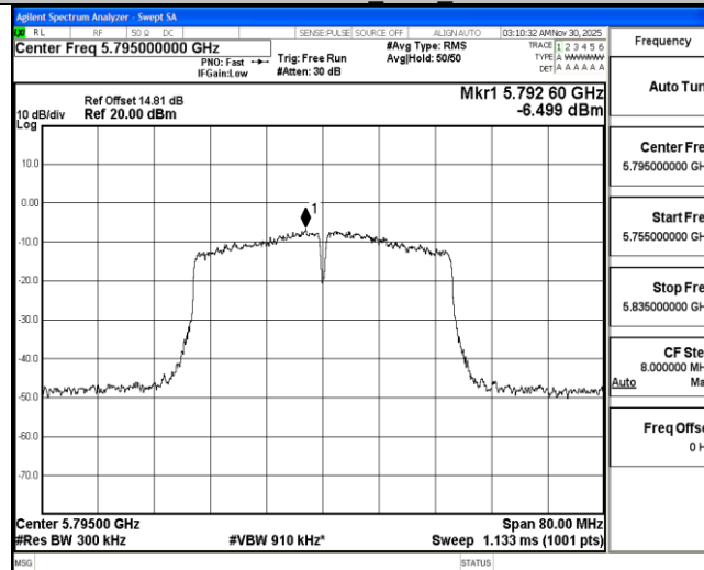
11N40MIMO Ant3 5795
