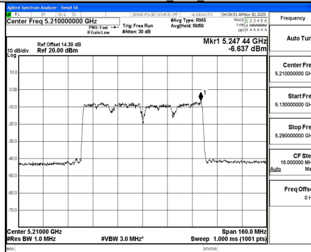
11AC80MIMO_Ant3_5210
