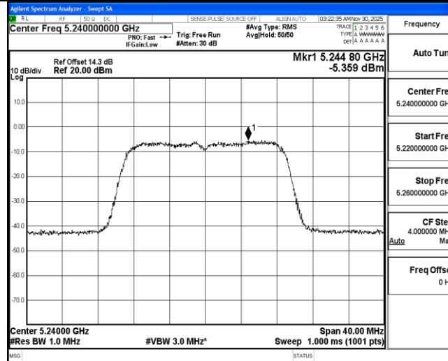
11AC20MIMO_Ant2_5240
