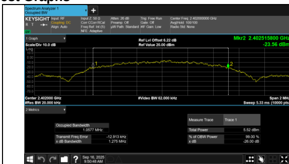
BLE 1M Channel 0
