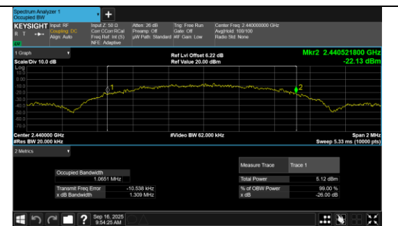
BLE 1M Channel 19
