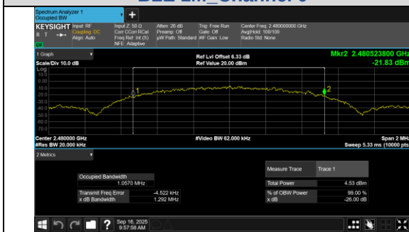
BLE 1M Channel 39
