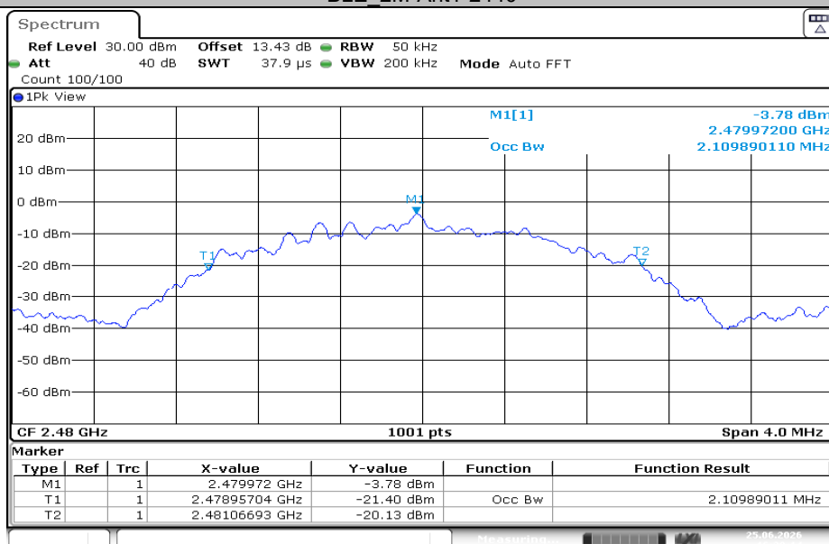
BLE_2M-Ant1-2480
