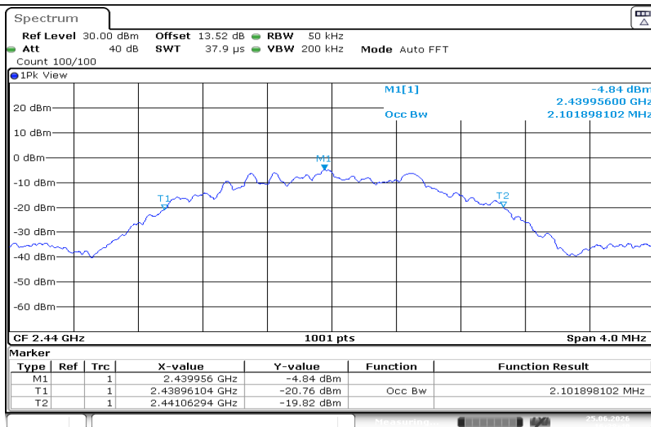
BLE_2M-Ant1-2440
