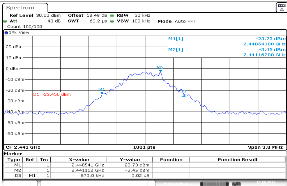
DH5-Ant1-2441
