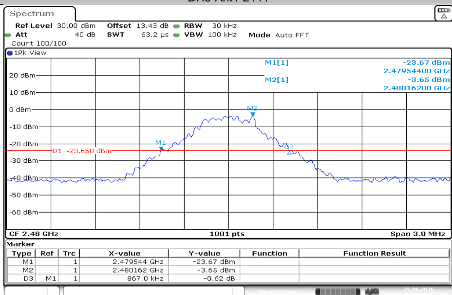
DH5-Ant1-2480
