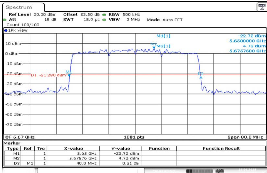
11AX40MIMO-Ant1-5670
