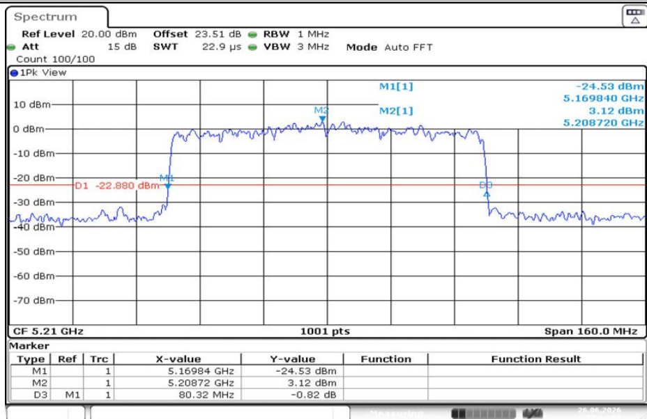
11AX80MIMO-Ant2-5210
