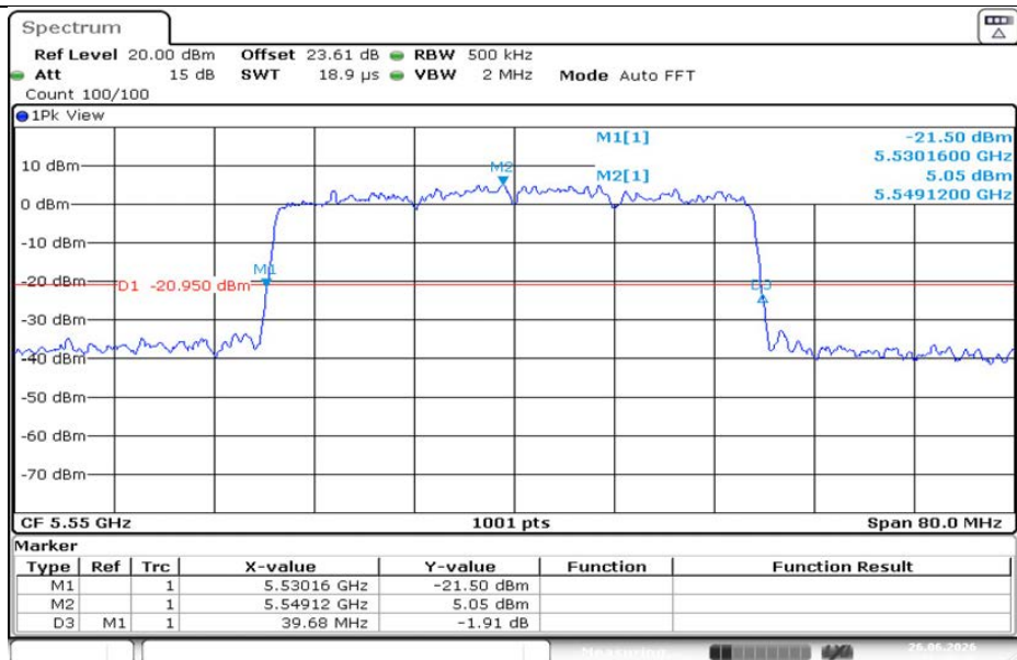
11AX40MIMO-Ant1-5550
