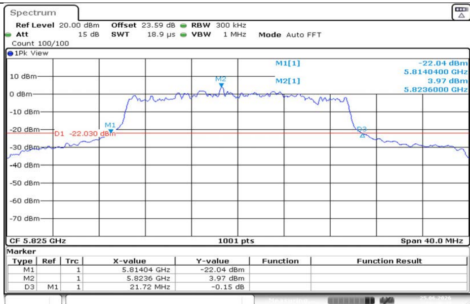
11AX20MIMO-Ant1-5825
