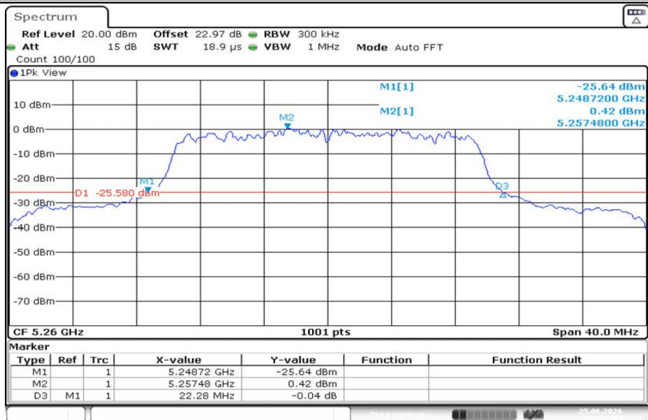
11AX20MIMO-Ant2-5260
