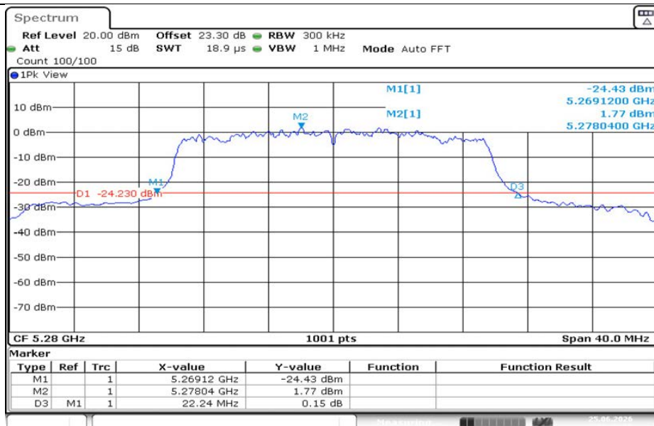
11AX20MIMO-Ant1-5280
