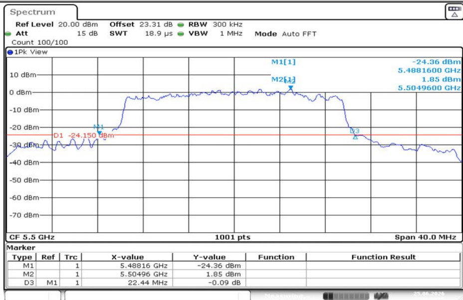
11AX20MIMO-Ant2-5500
