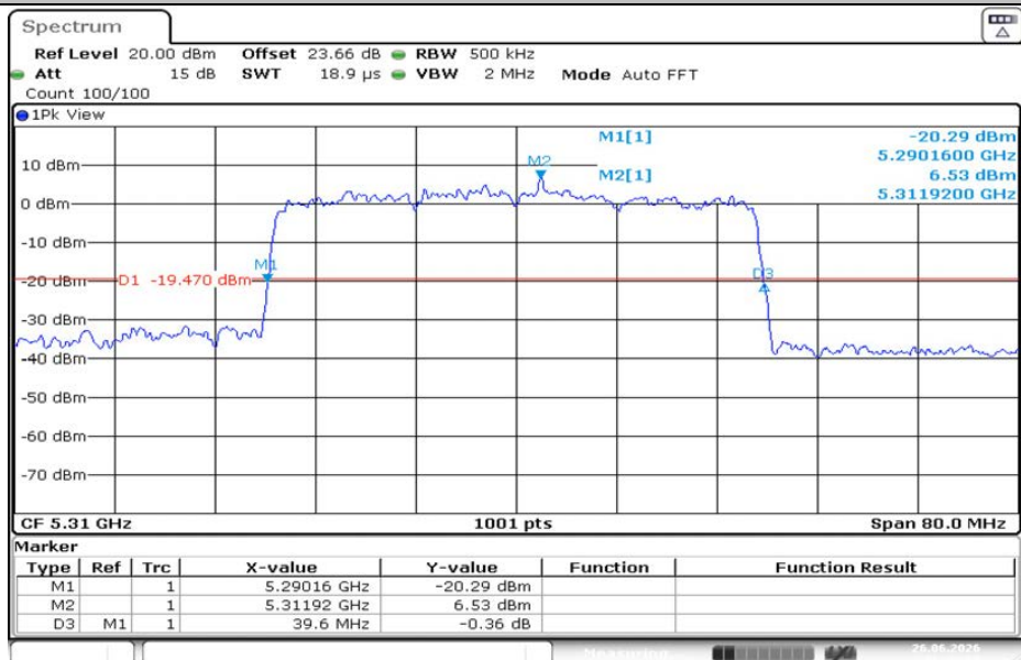
11AX40MIMO-Ant2-5310
