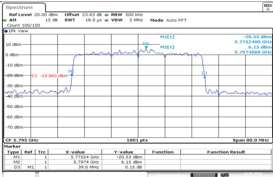
11AX40MIMO-Ant1-5795
