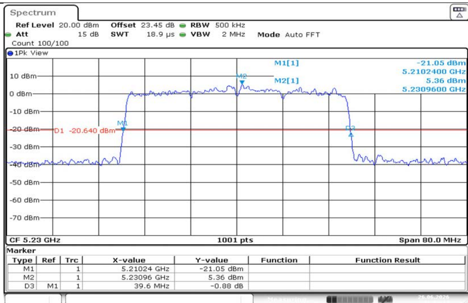
11AX40MIMO-Ant1-5230
