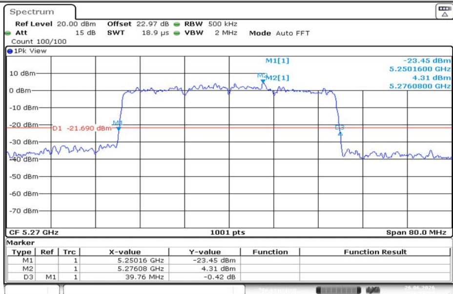
11AX40MIMO-Ant2-5270
