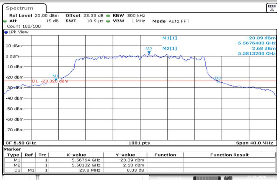
11AX20MIMO-Ant1-5580
