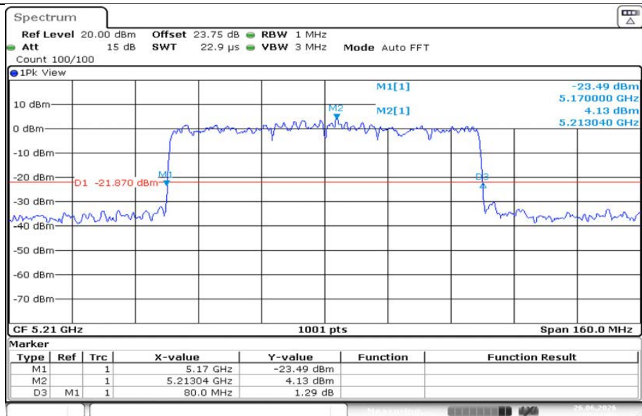
11AX80MIMO-Ant1-5210
