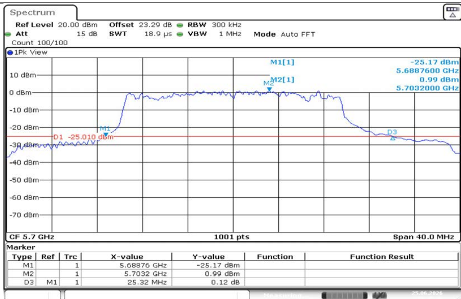
11AX20MIMO-Ant1-5700
