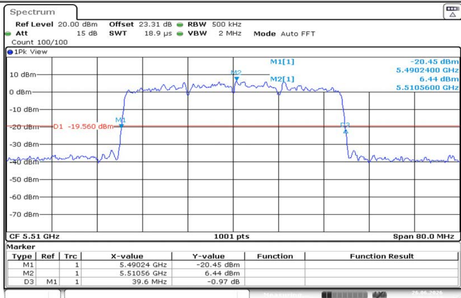
11AX40MIMO-Ant2-5510
