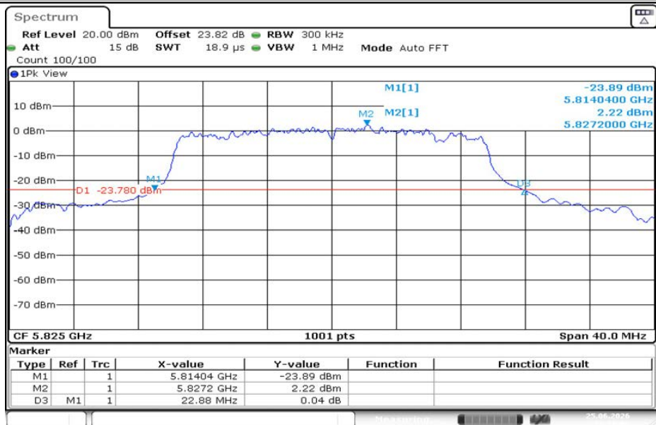
11AX20MIMO-Ant2-5825
