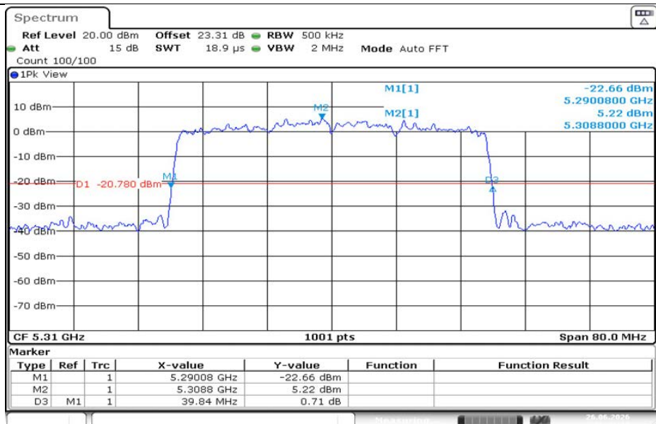
11AX40MIMO-Ant1-5310
