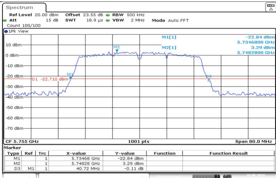
11AC40MIMO-Ant1-5755
