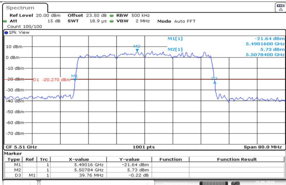
11AX40MIMO-Ant1-5510
