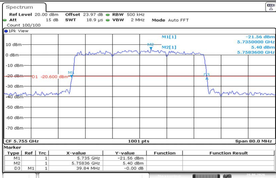
11AX40MIMO-Ant2-5755
