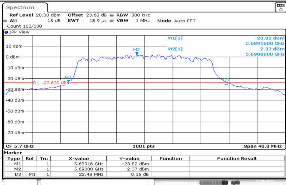
11AX20MIMO-Ant2-5700
