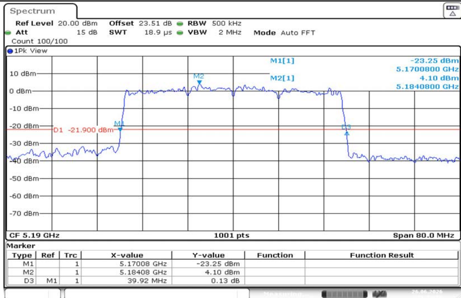
11AX40MIMO-Ant2-5190
