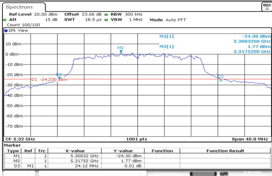
11AX20MIMO-Ant2-5320
