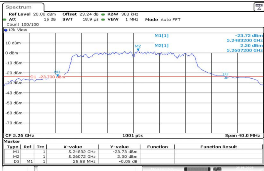
11AX20MIMO-Ant1-5260
