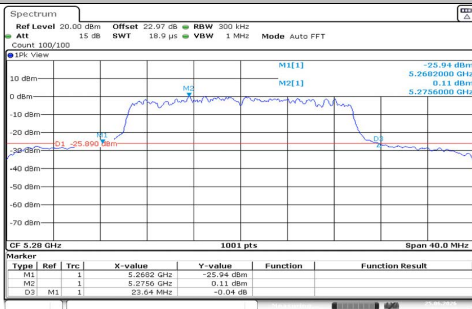
11AX20MIMO-Ant1-5280
