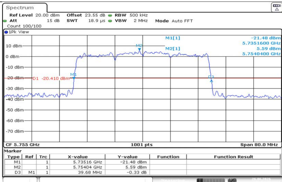
11AX40MIMO-Ant1-5755
