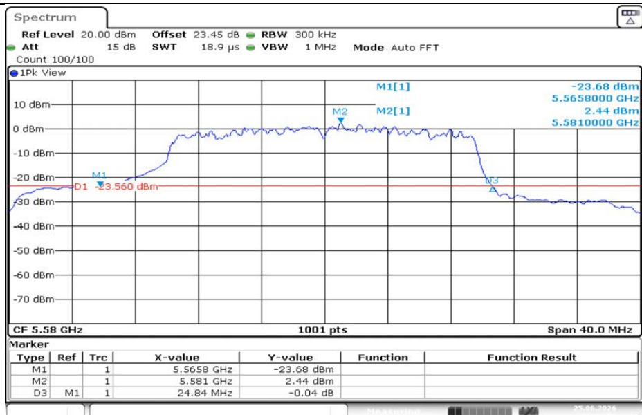
11AX20MIMO-Ant1-5580
