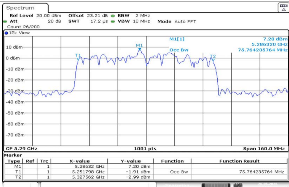
11AC80MIMO-Ant1-5290
