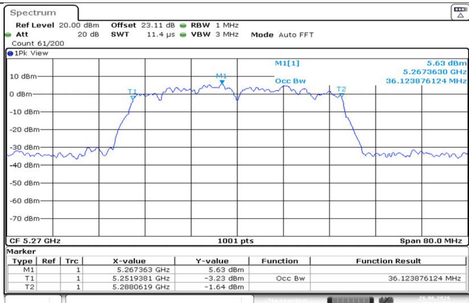
11AC40MIMO-Ant1-5270
