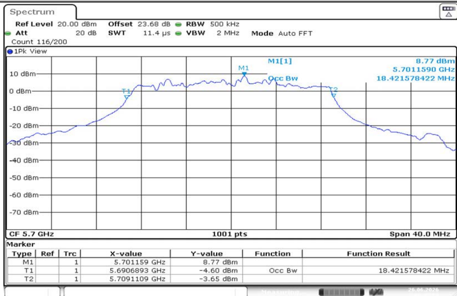
11N20MIMO-Ant2-5700
