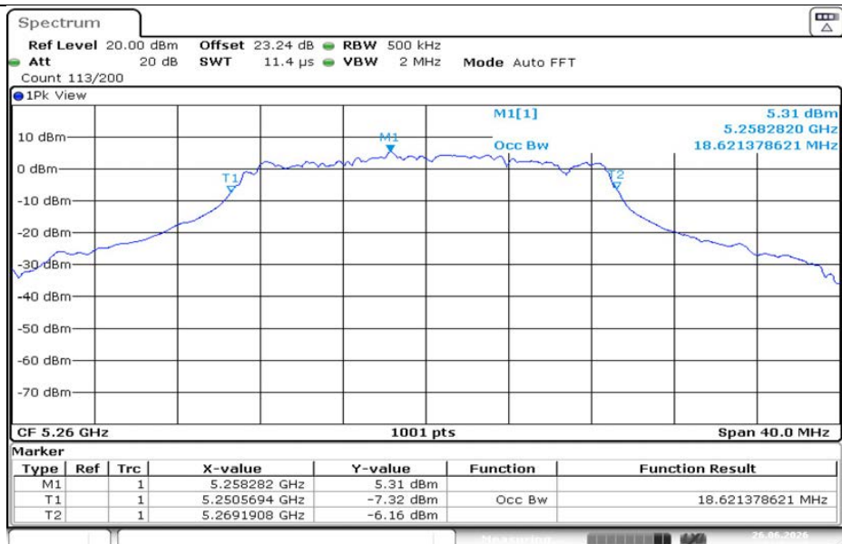
11AC20MIMO-Ant1-5260
