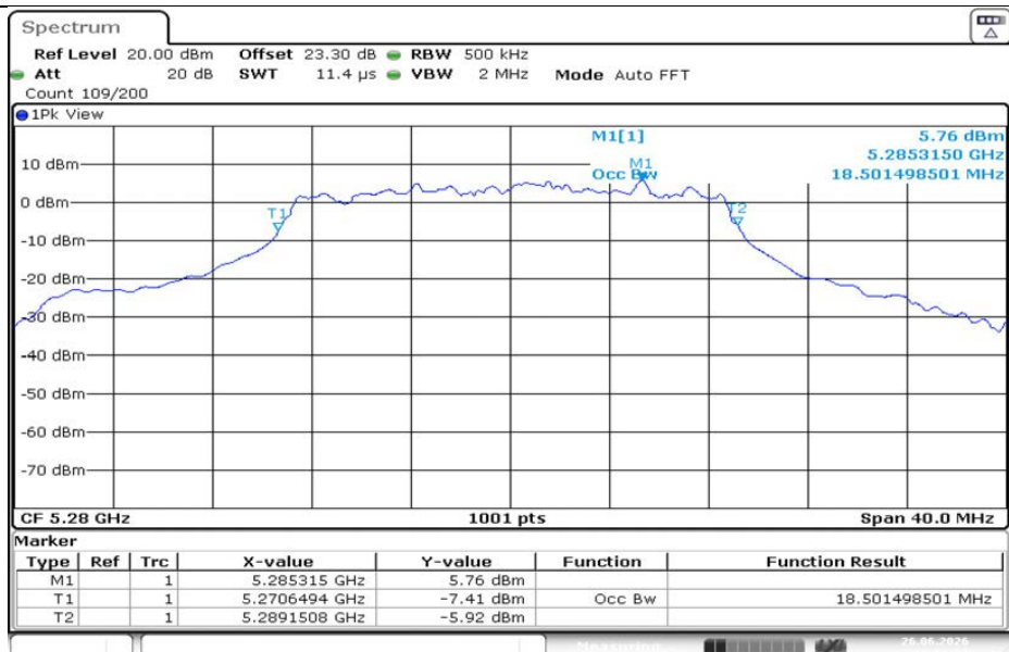
11N20MIMO-Ant1-5280
