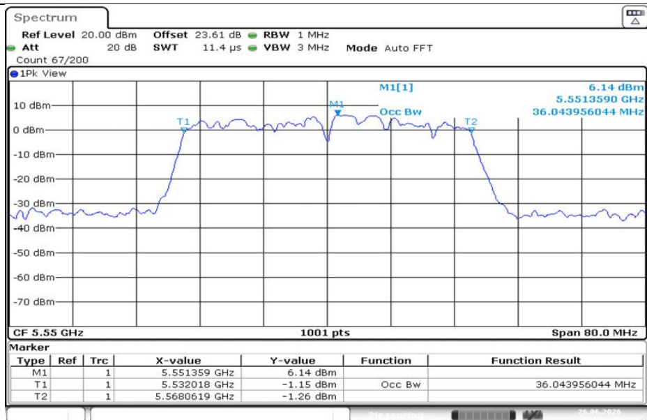
11AC40MIMO-Ant1-5550
