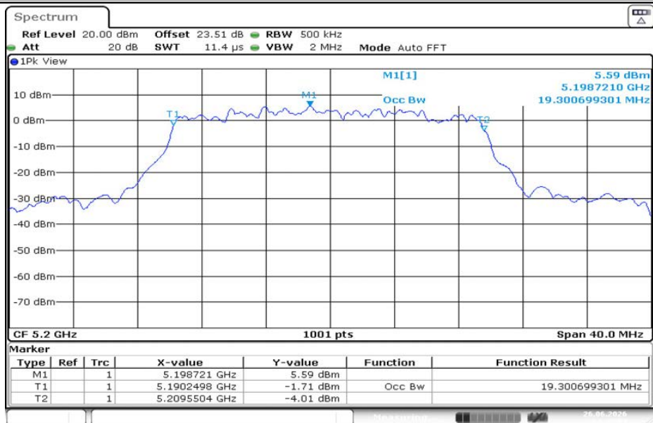
11AX20MIMO-Ant2-5200
