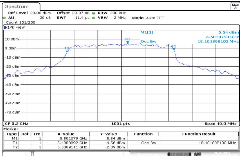
11N20MIMO-Ant1-5500
