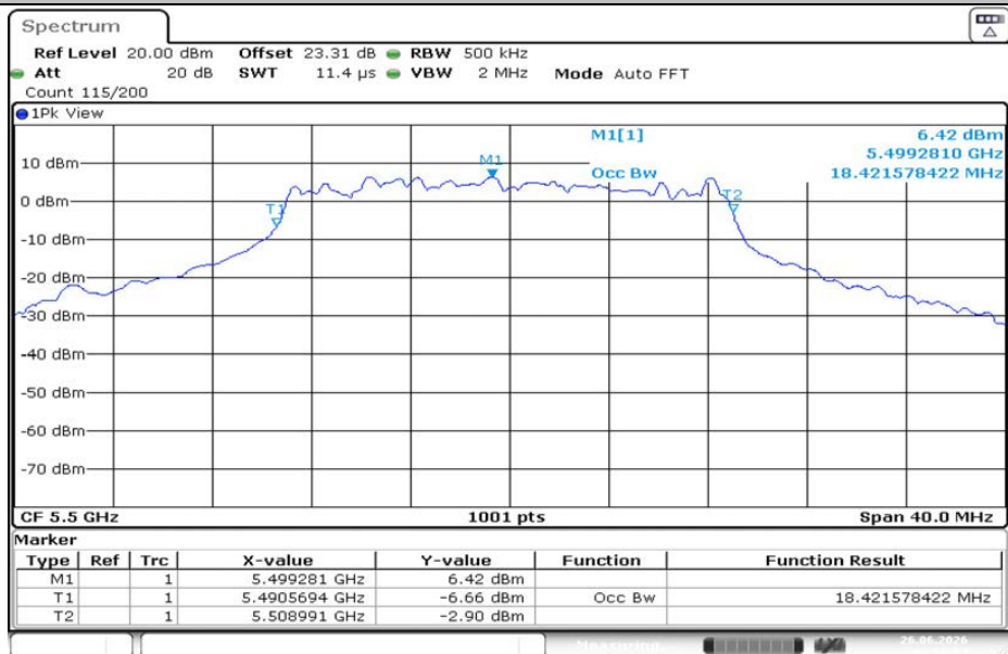
11N20MIMO-Ant2-5500
