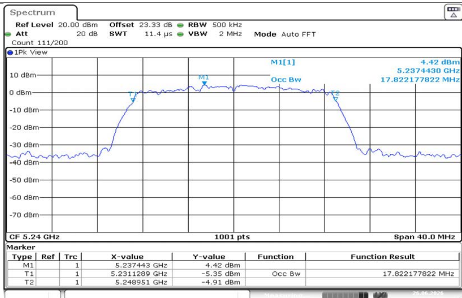
11N20MIMO-Ant1-5240
