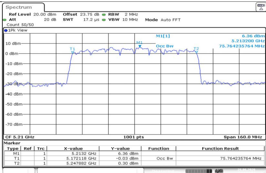
11AC80MIMO-Ant1-5210
