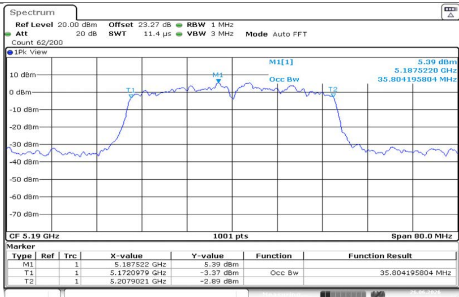
11N40MIMO-Ant1-5190
