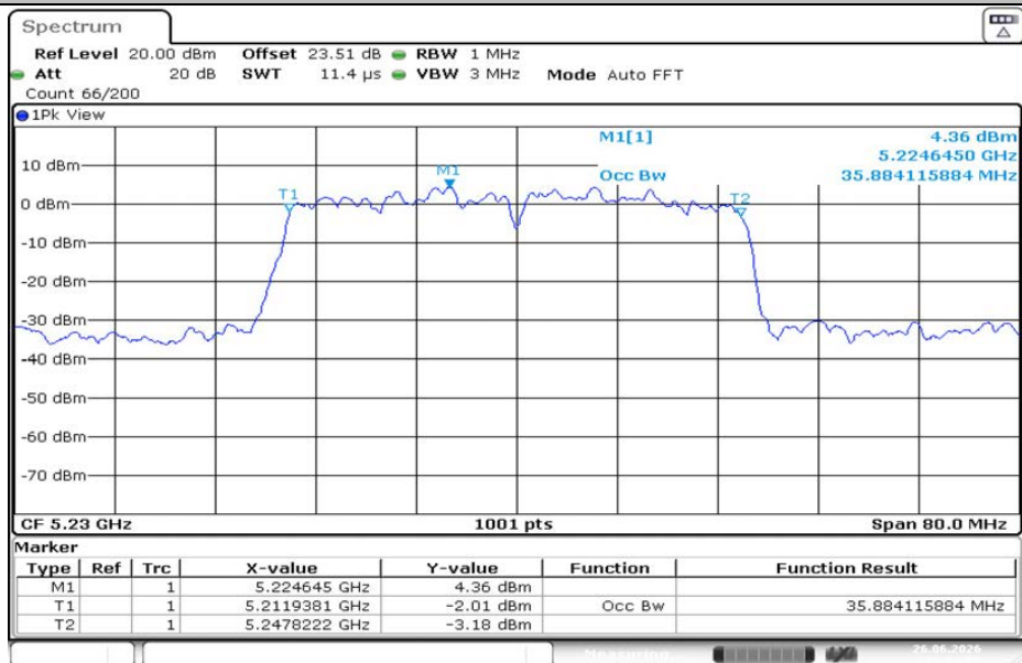
11N40MIMO-Ant2-5230
