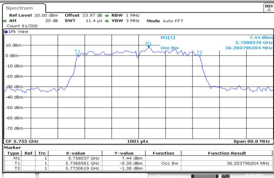
11N40MIMO-Ant1-5755
