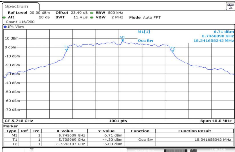
11N20MIMO-Ant1-5745
