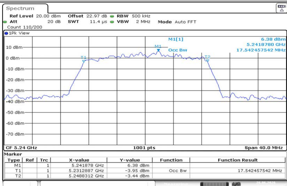
11N20MIMO-Ant1-5240
