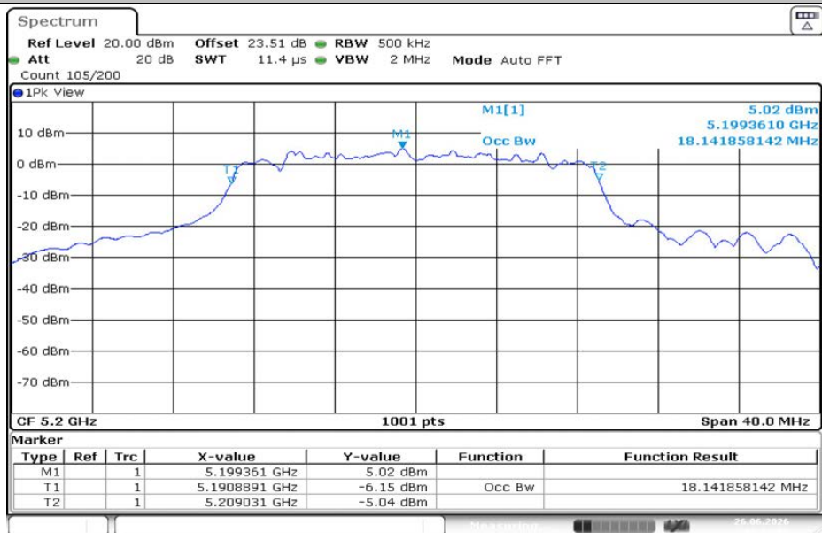
11N20MIMO-Ant2-5200
