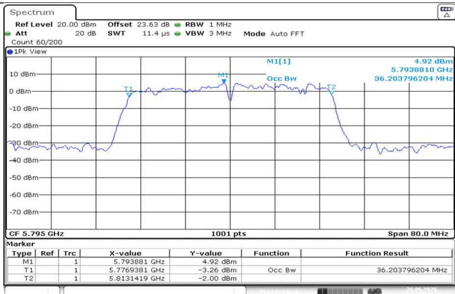
11AC40MIMO-Ant1-5795
