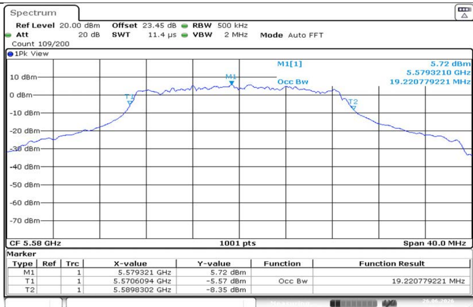
11N20MIMO-Ant1-5580
