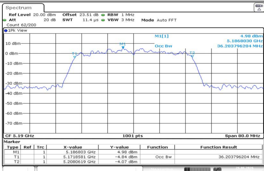
11N40MIMO-Ant1-5190
