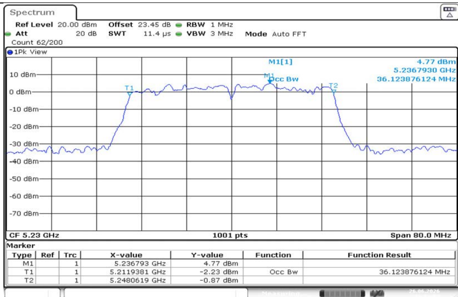
11N40MIMO-Ant1-5230
