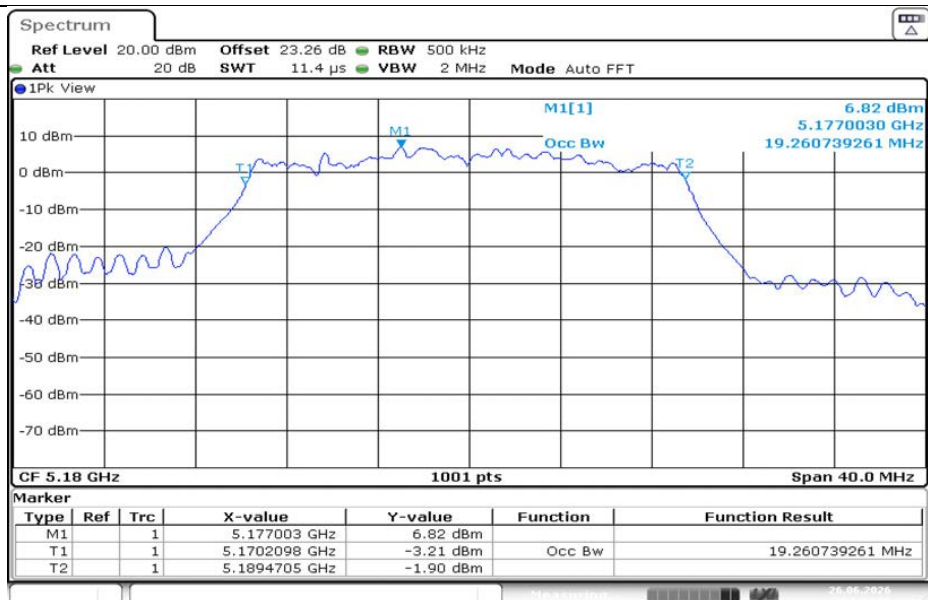
11AX20MIMO-Ant1-5180
