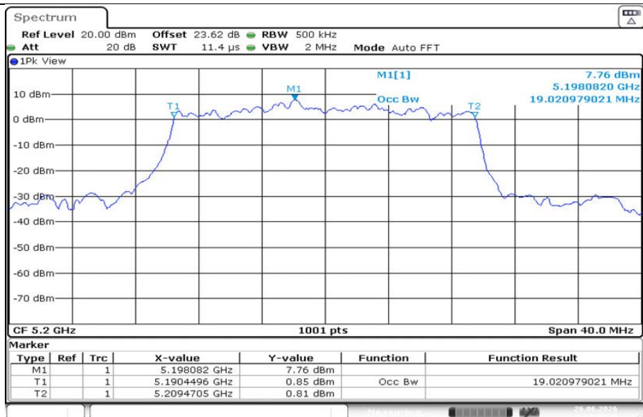
11AX20MIMO-Ant1-5200
