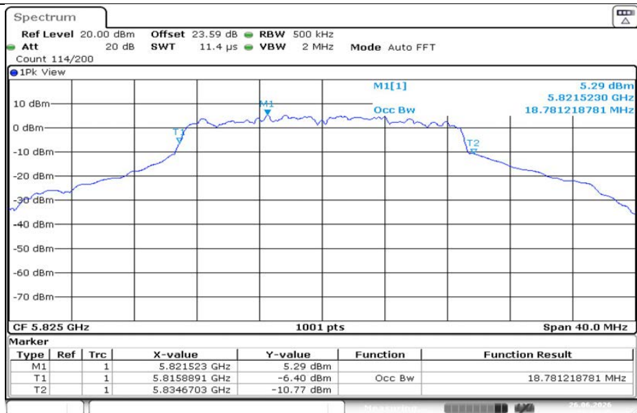
11N20MIMO-Ant1-5825
