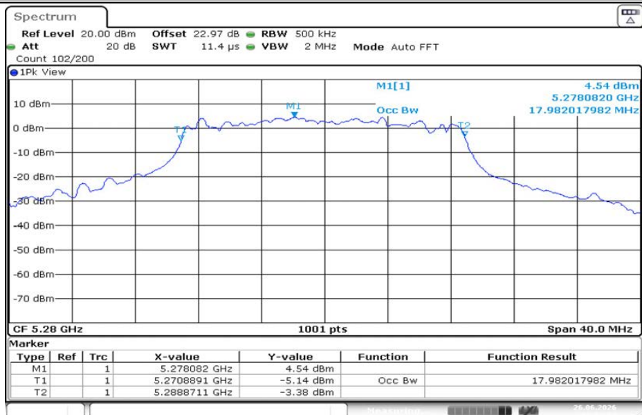
11N20MIMO-Ant2-5280
