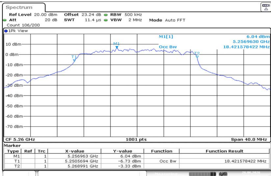
11N20MIMO-Ant1-5260
