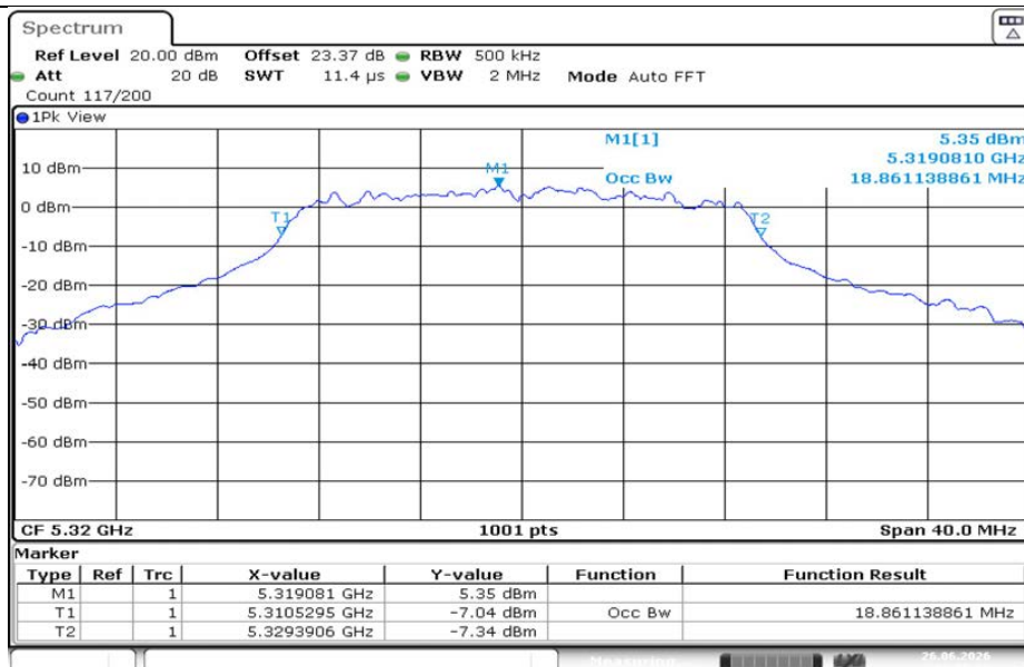
11N20MIMO-Ant1-5320
