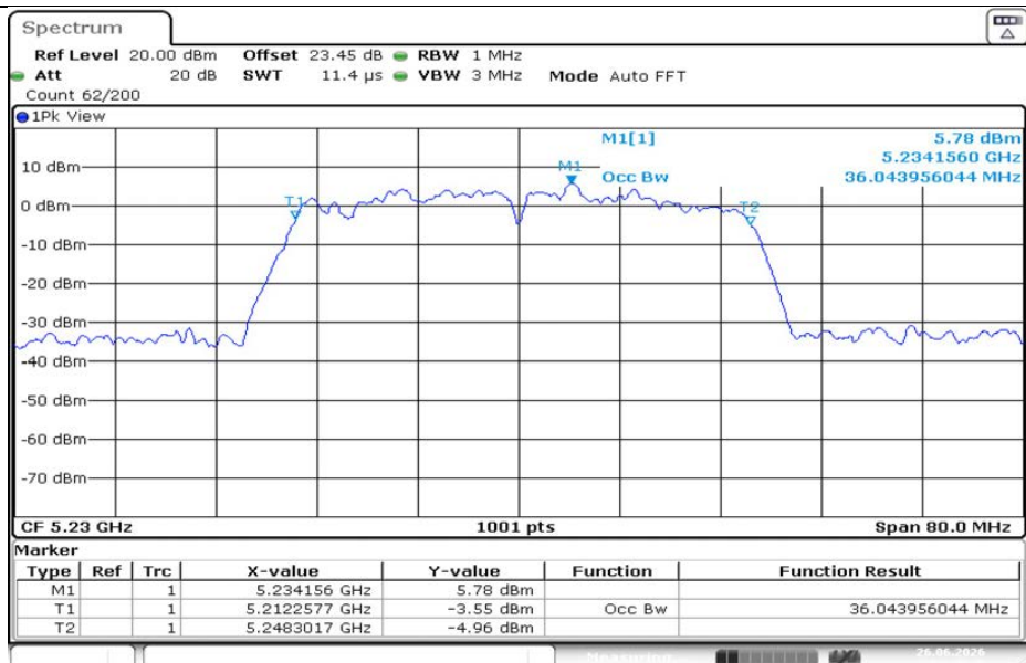
11AC40MIMO-Ant1-5230
