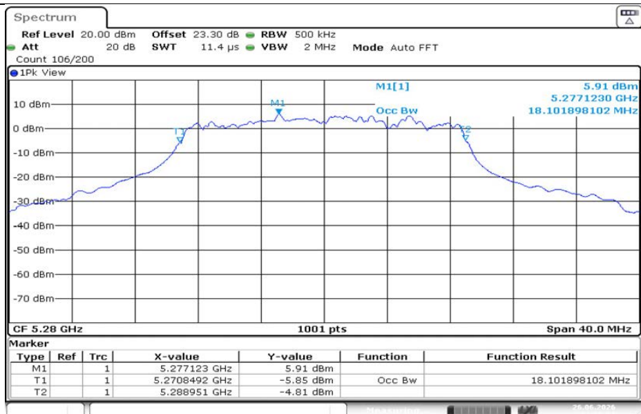
11AC20MIMO-Ant1-5280
