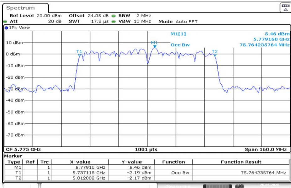
11AC80MIMO-Ant1-5775
