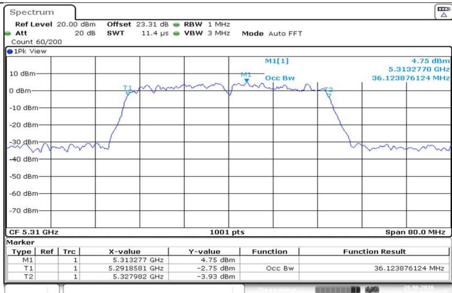
11N40MIMO-Ant1-5310
