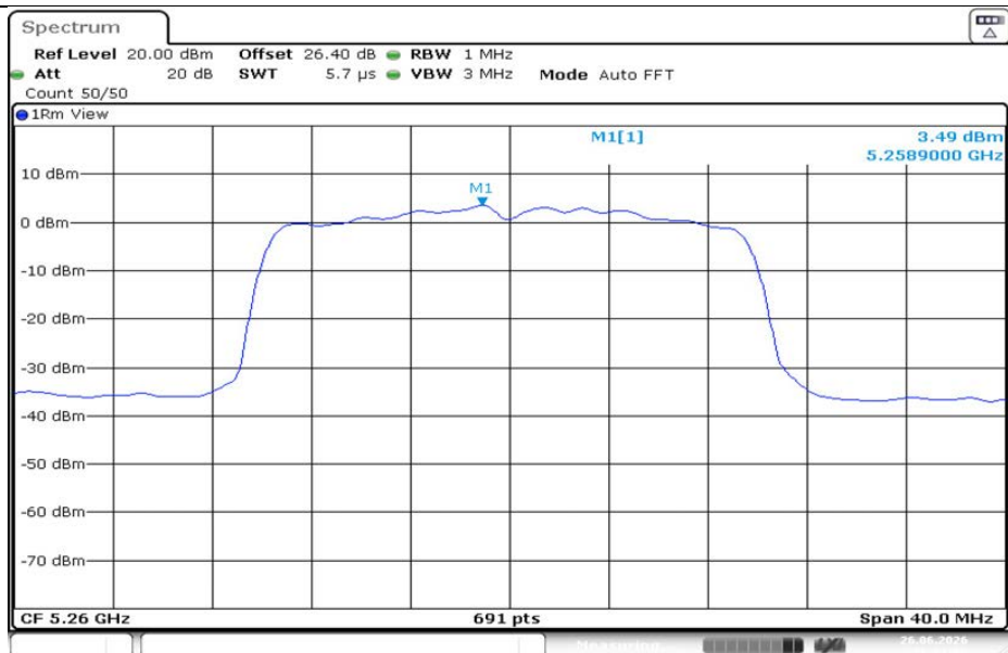
11AX20MIMO-Ant1-5260-PASS
