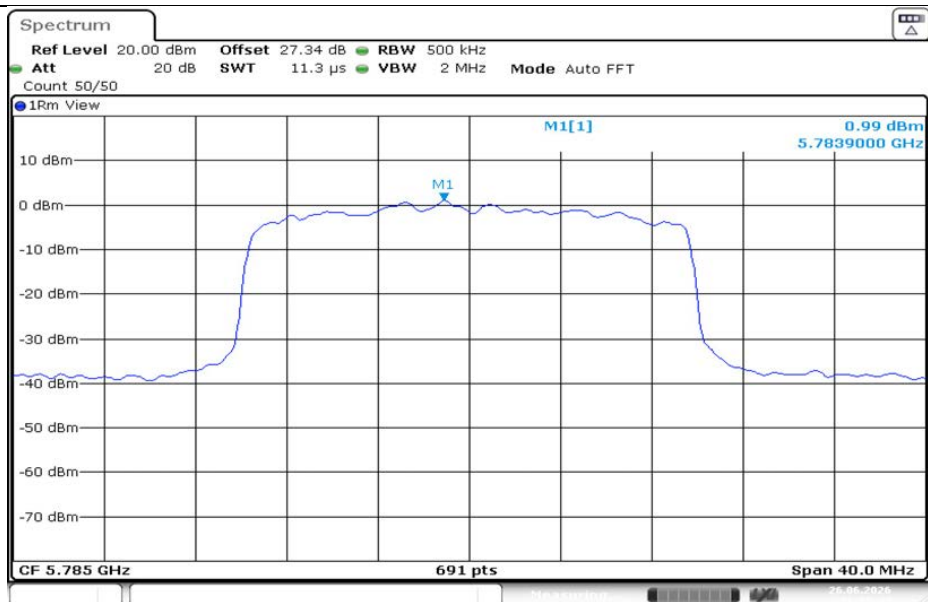
11AX20MIMO-Ant1-5785-PASS
