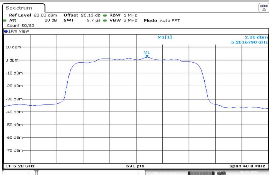
11AX20MIMO-Ant1-5280-PASS
