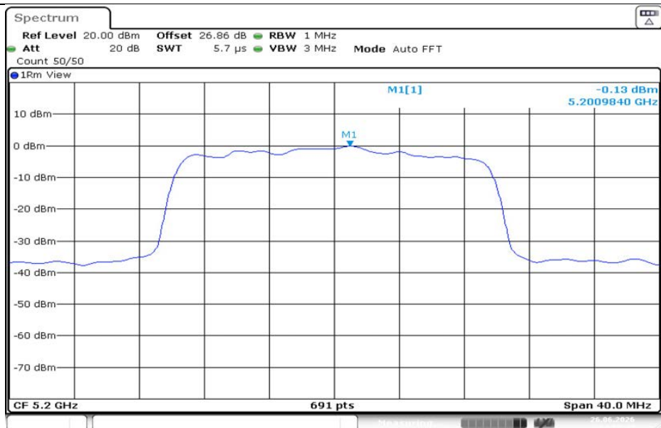
11AX20MIMO-Ant1-5200-PASS
