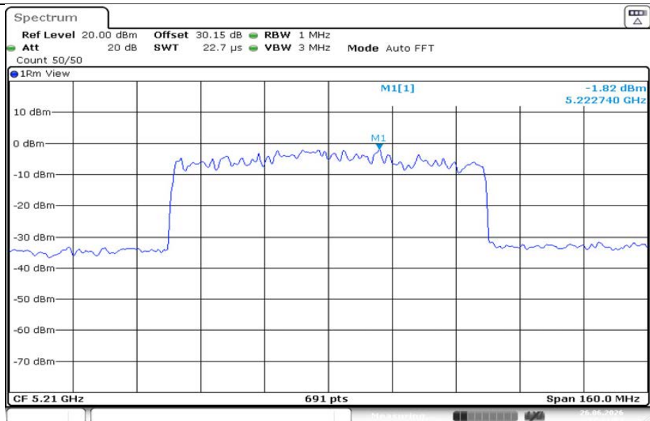
11AX80MIMO-Ant1-5210-PASS
