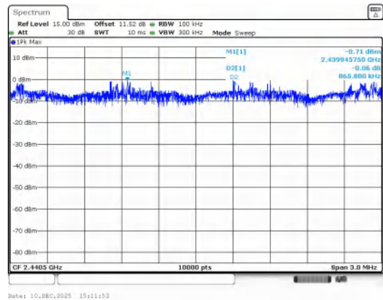
π/4DQPSK
