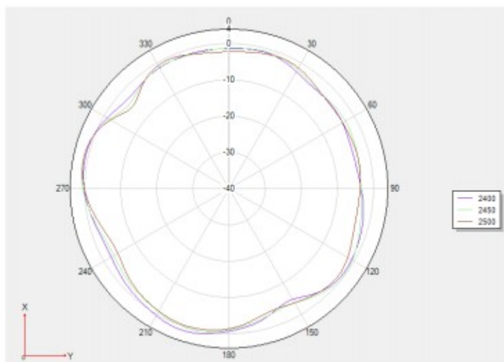
Theta 90 2D 图
