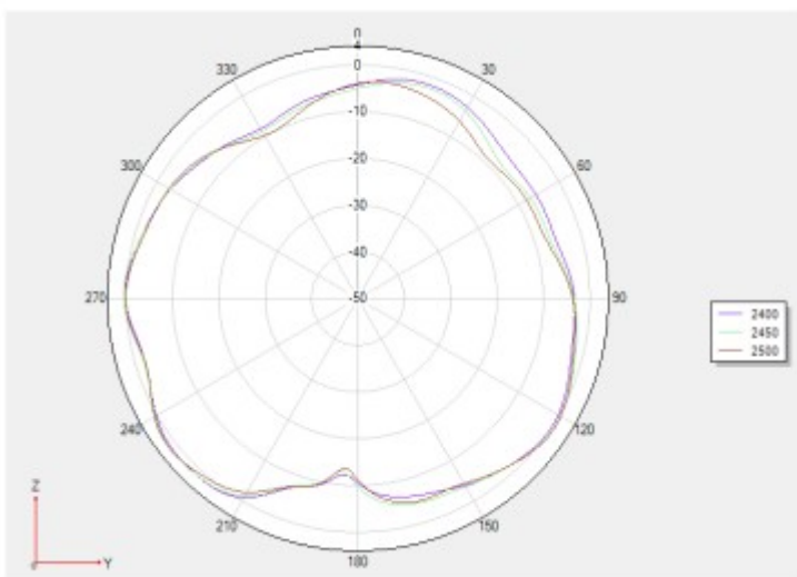
Theta 90 2D 图
