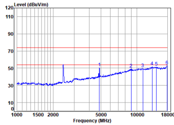
11n_40M_TX_CH_06_Horizontal
