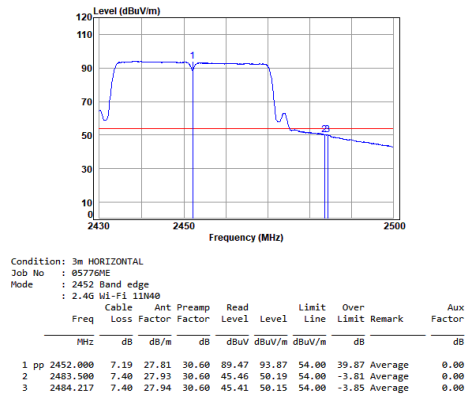
11n_HT(40M)_TX_CH_09_Horizontal-Avg
