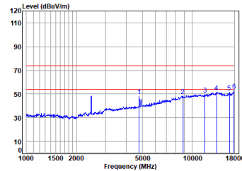
11b_TX_CH_11_Vertical
