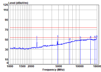
11b_TX_CH_06_Vertical
