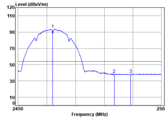
11b_TX_CH_11_Vertical-Avg
