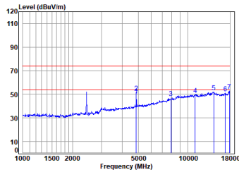
11b_TX_CH_06_Horizontal
