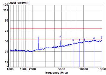
11g_TX_CH_01_Horizontal
