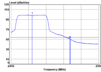
11g_TX_CH_11_Horizontal-Avg
