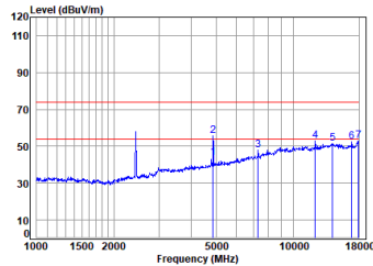
11g_TX_CH_06_Horizontal
