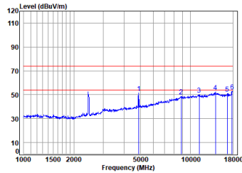
11n_40M_TX_CH_09_Horizontal
