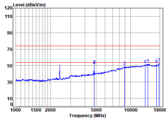
11b_TX_CH_01_Horizontal
