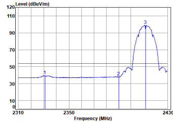
11b_TX_CH_01_Horizontal-Avg
