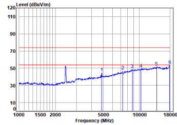
11n_40M_TX_CH_06_Vertical
