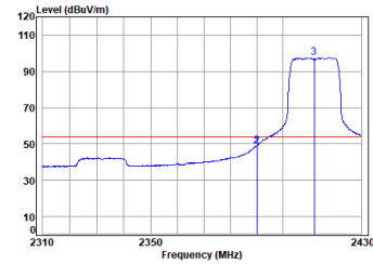
11n_HT(20M)_TX_CH_01_Horizontal-Avg
