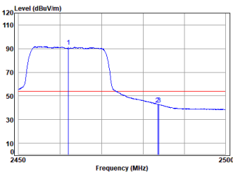
11n_HT(20M)_TX_CH_11_Vertical-Avg
