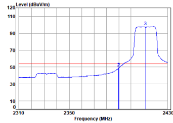
11g_TX_CH_01_Horizontal-Avg
