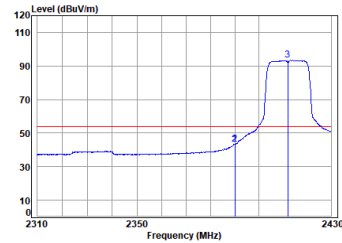
11g_TX_CH_01_Vertical-Avg
