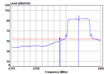
11n_HT(40M)_TX_CH_03_Horizontal-Avg
