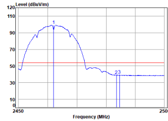
11b_TX_CH_11_Horizontal-Avg
