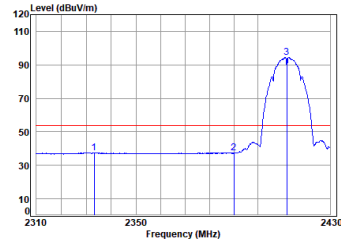
11b_TX_CH_01_Vertical-Avg
