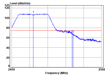
11n_HT(20M)_TX_CH_11_Horizontal-Peak
