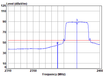
11n_HT(40M)_TX_CH_03_Vertical-Avg
