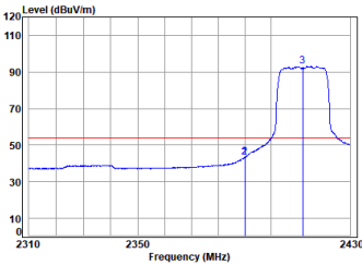
11n_HT(20M)_TX_CH_01_Vertical-Avg
