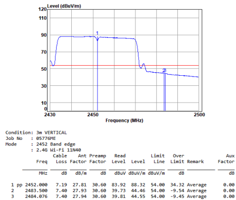
11n_HT(40M)_TX_CH_09_Vertical-Avg
