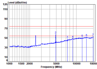
11g_TX_CH_11_Horizontal
