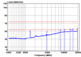
11n_40M_TX_CH_09_Vertical
