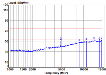
11b_TX_CH_11_Horizontal
