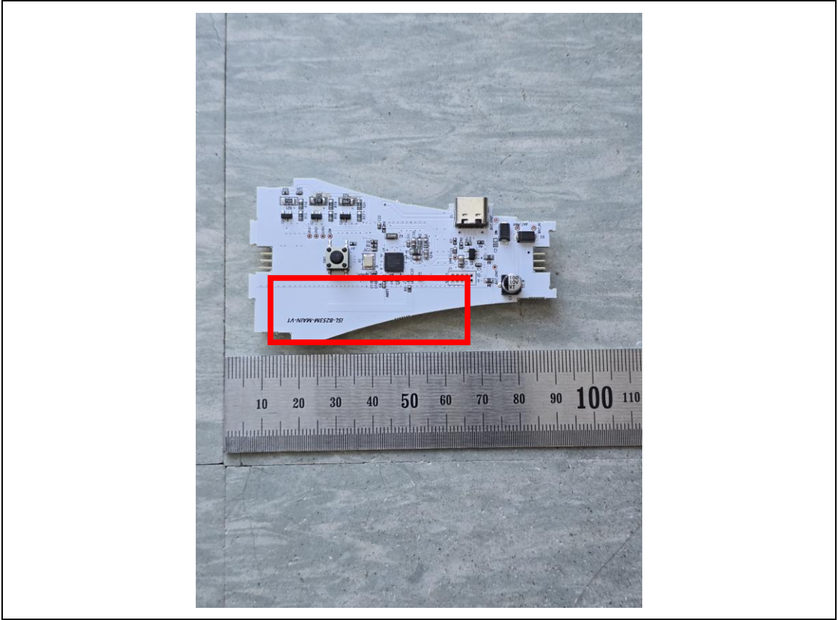
Antenna(2.4 GHz)
