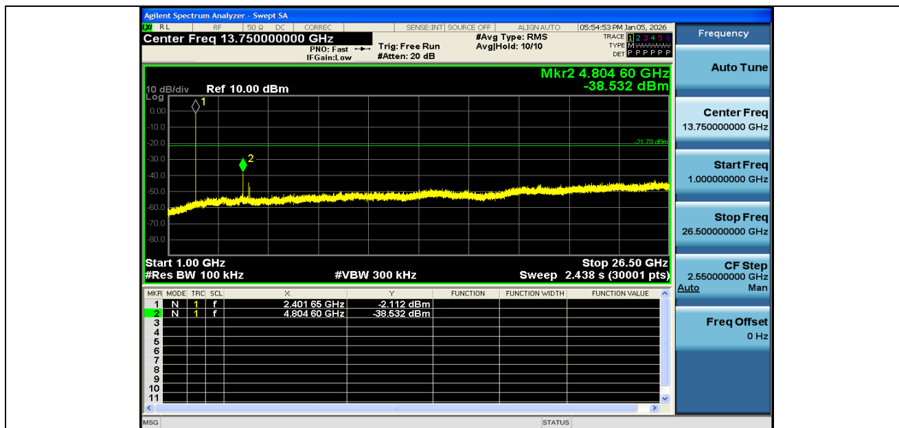
BLE 1M-Ant1-2402-1000~26500-PASS
