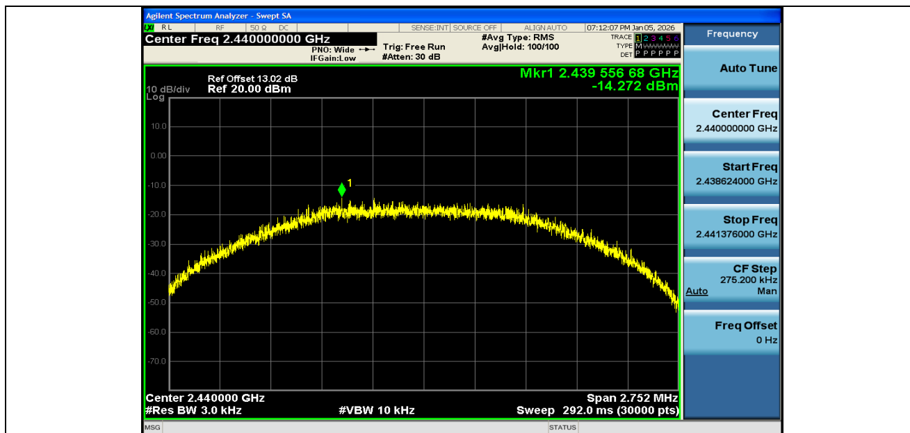
BLE 2M-Ant1-2440-PASS
