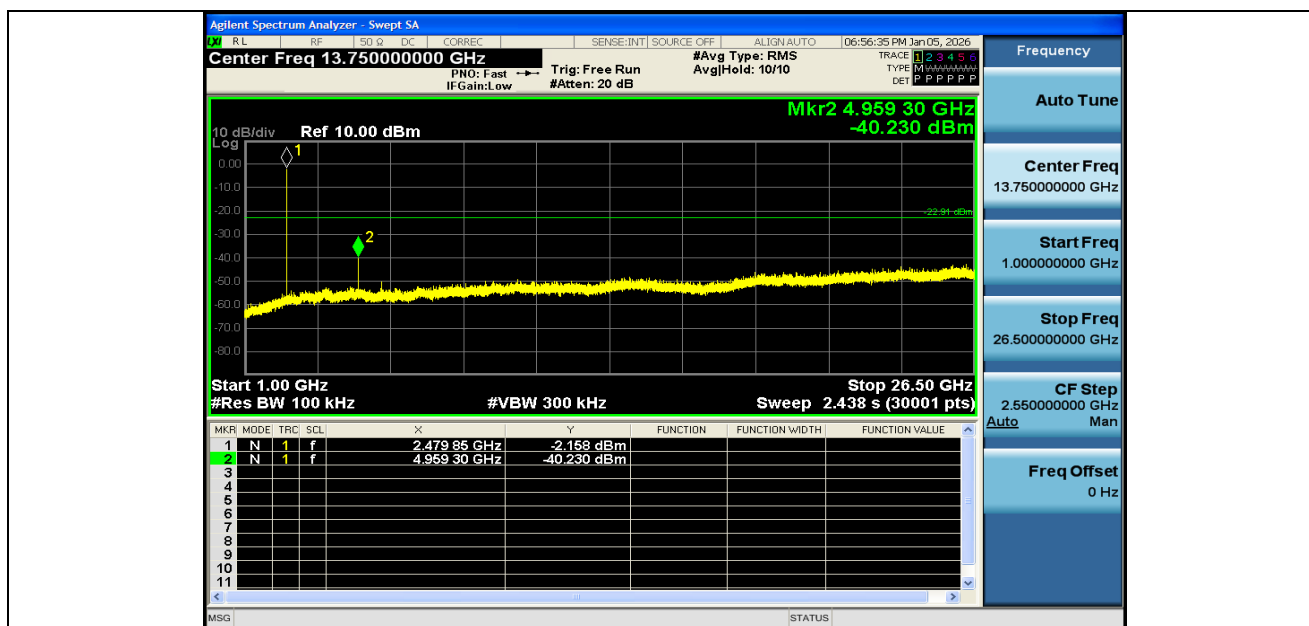
BLE 1M-Ant1-2480-1000~26500-PASS
