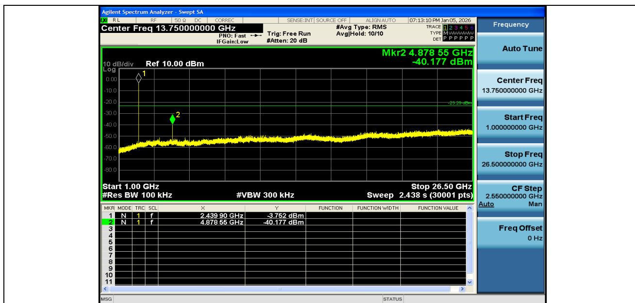
BLE 2M-Ant1-2440-1000~26500-PASS
