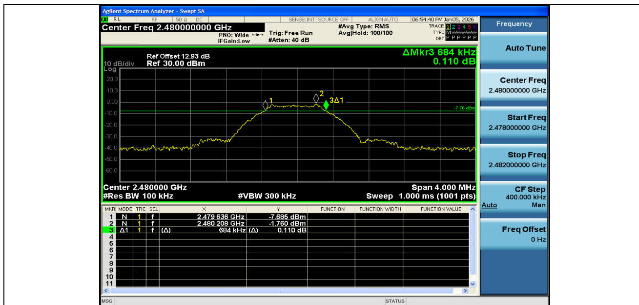
BLE 1M-Ant1-2480-PASS
