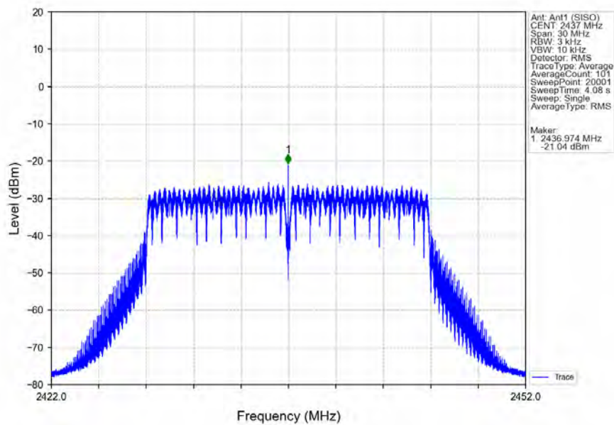
802.11n(HT20)_MCH_2437MHz_Ant1 (SISO)_NTNV
