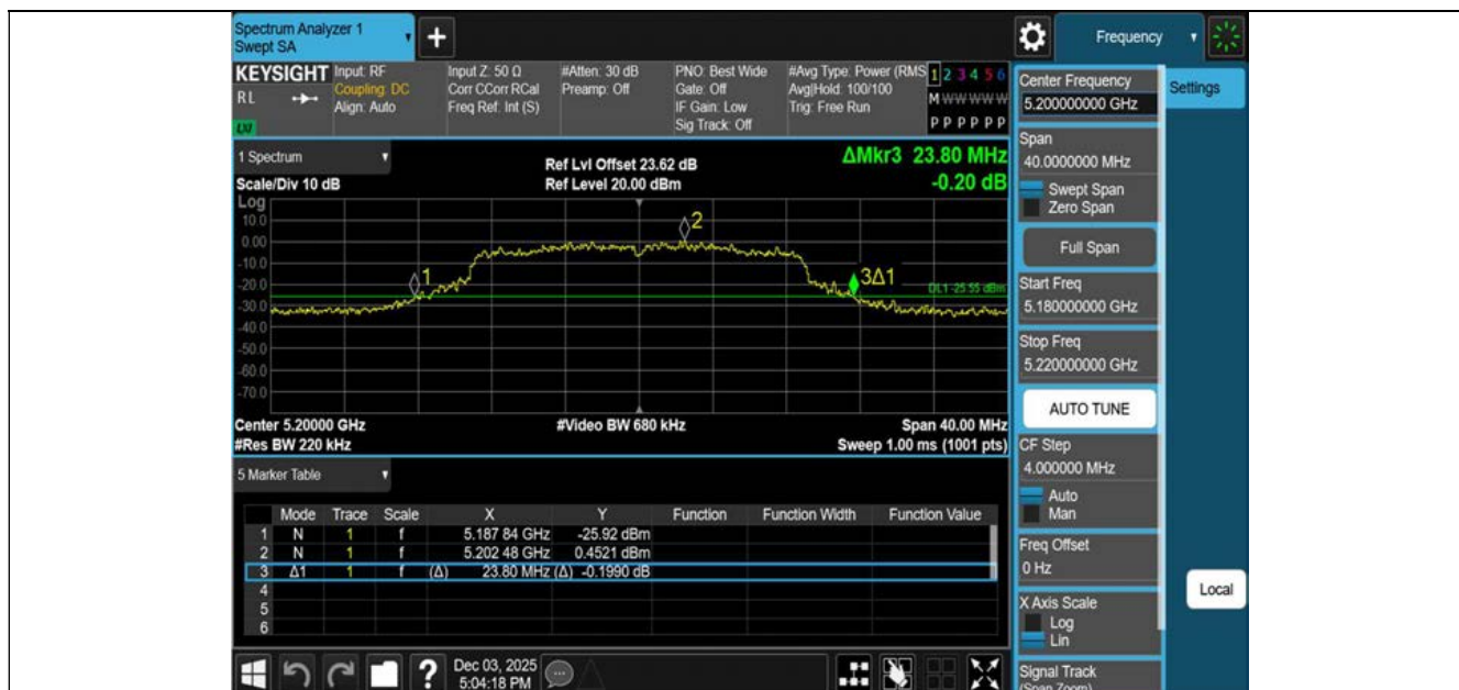
11AC20MIMO-Ant1-5200
