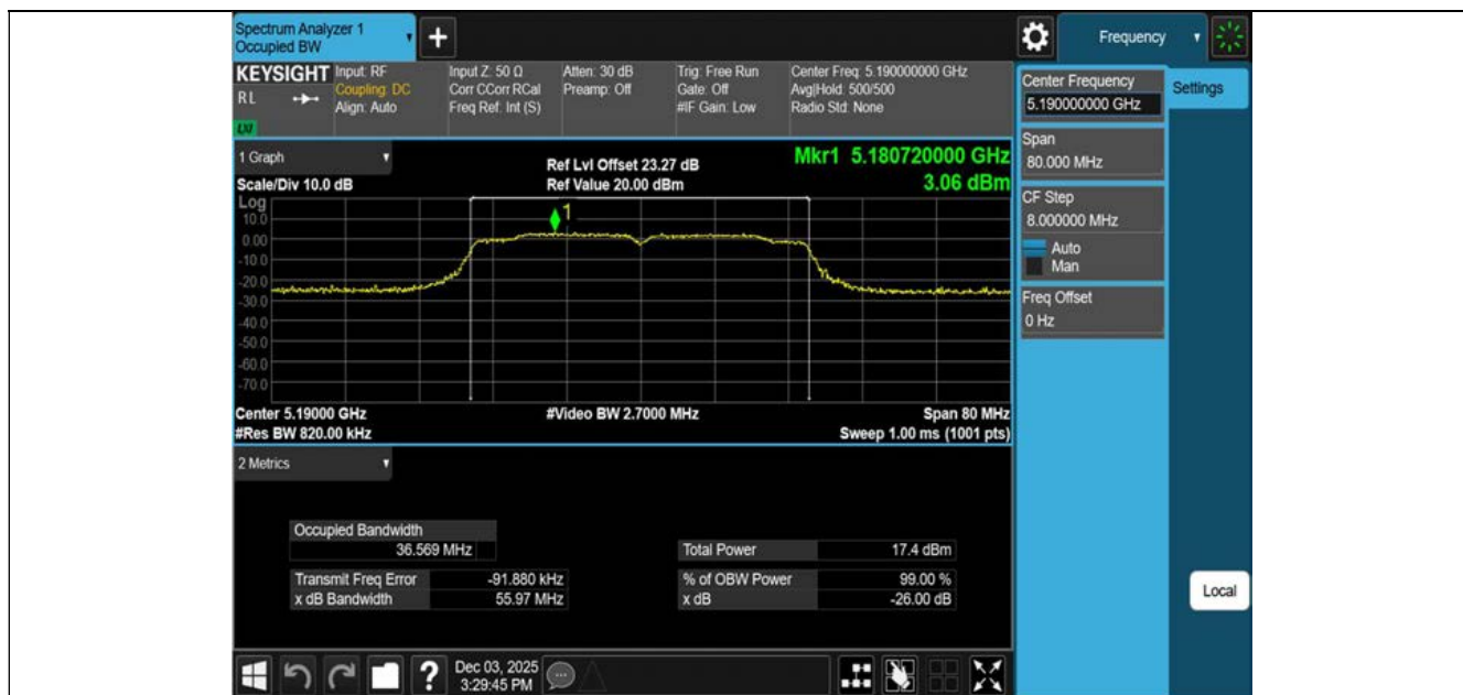
11N40MIMO-Ant1-5190
