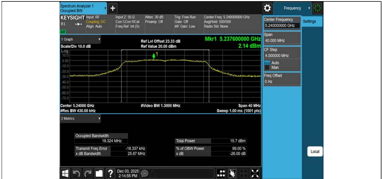
11N20MIMO-Ant1-5240
