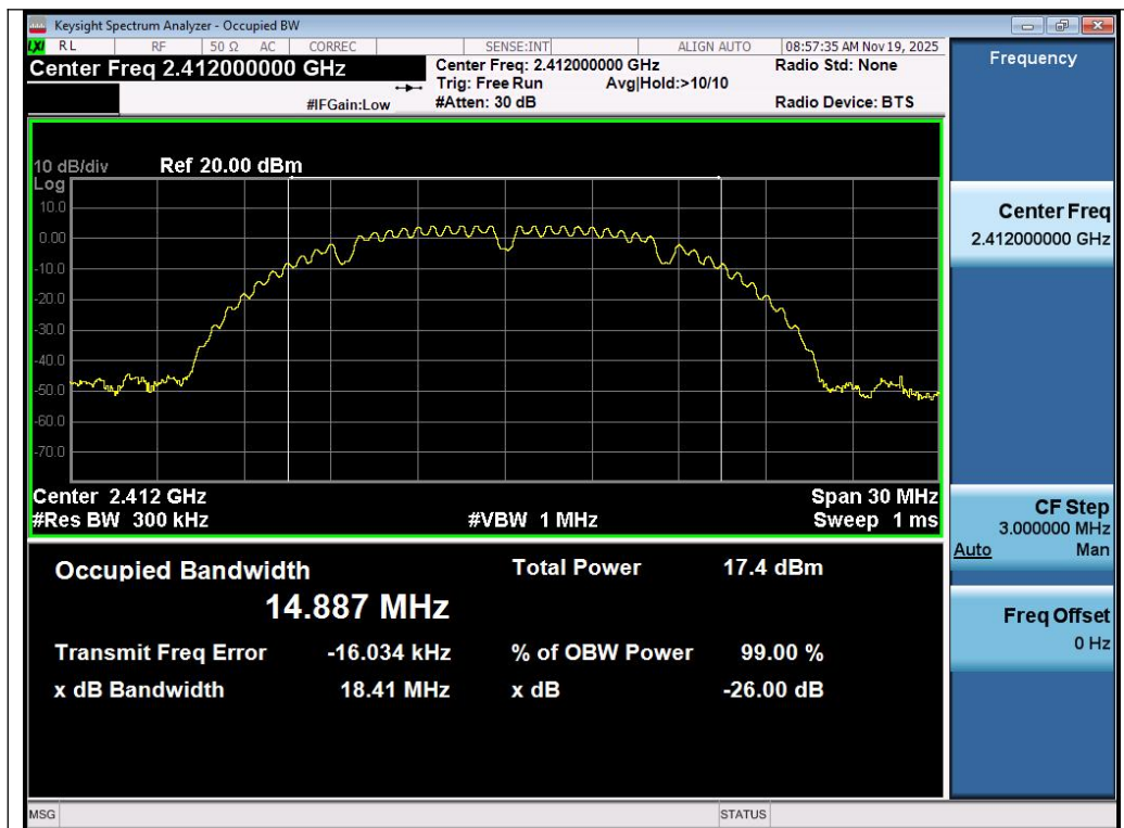
Test_Graph_802.11b_Chain A_2412_1Mbps_OBW
