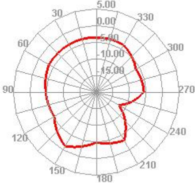
2410.000MHz E2
