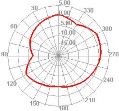
2410.000MHz E1
