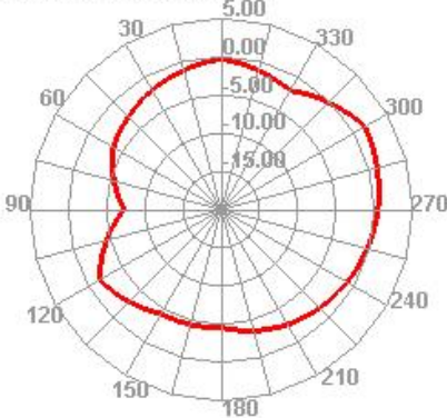
2410.000MHz
