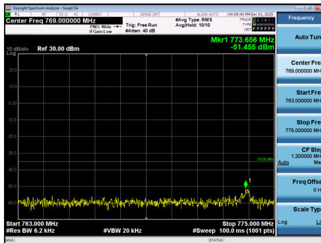
Band13-5MHz-QPSK-23255-1RB#0-Range3:763~775MHz
