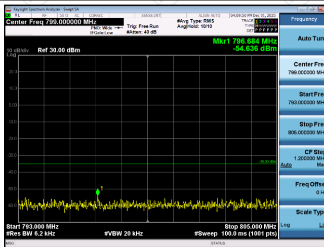
Band13-5MHz-QPSK-23255-1RB#0-Range4:793~805MHz
