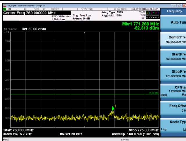
Band13-5MHz-QPSK-23230-1RB#0-Range3:763~775MHz
