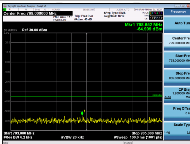
Band13-5MHz-QPSK-23230-1RB#0-Range4:793~805MHz
