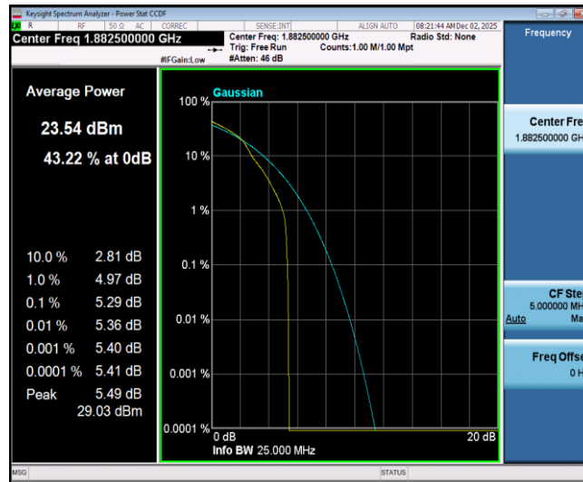
Band25-20MHz-16QAM-26365-1RB#0
