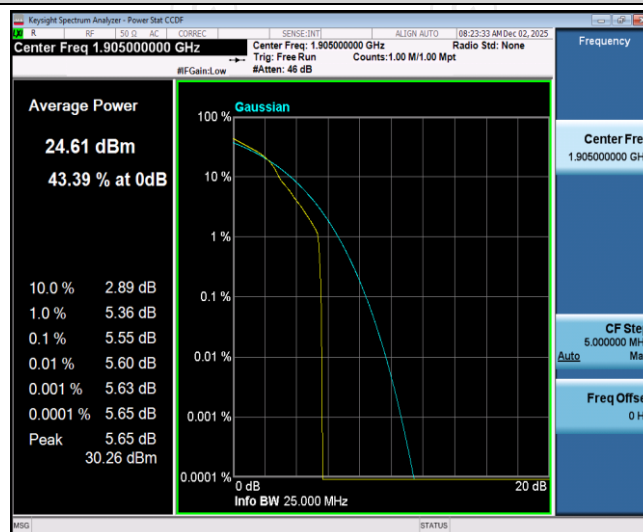
Band25-20MHz-16QAM-26590-1RB#0
