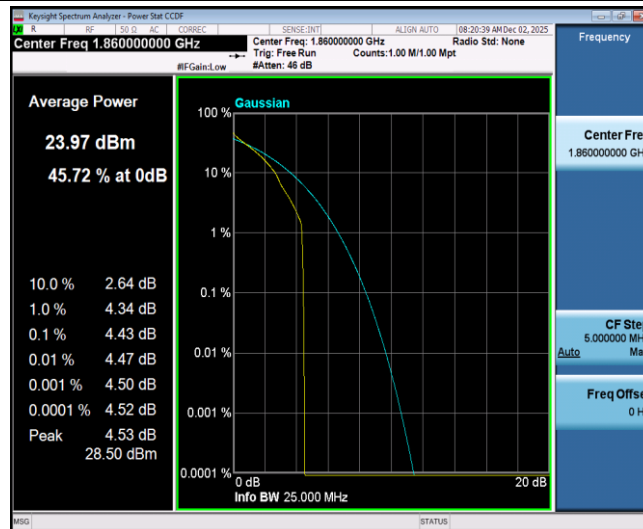
Band25-20MHz-QPSK-26140-1RB#0
