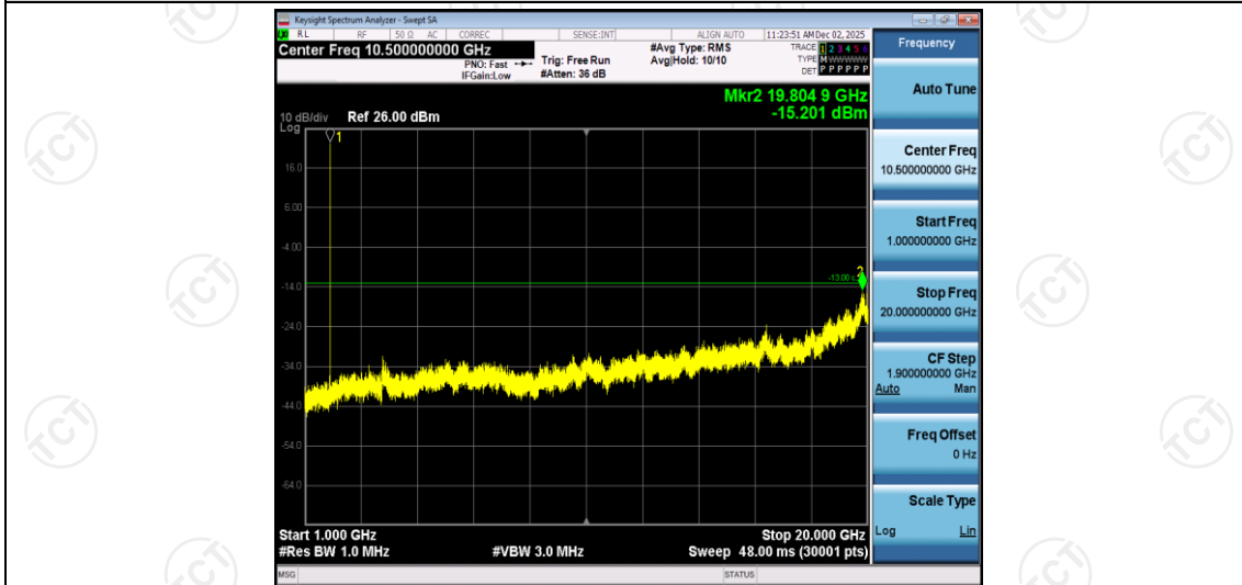
Band25-1.4MHz-QPSK-26047-1RB#0-Range2:1000~20000MHz
