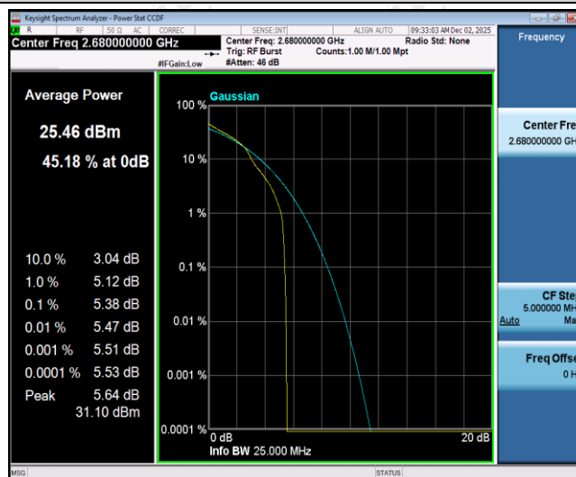
Band41-20MHz-16QAM-41490-1RB#0
