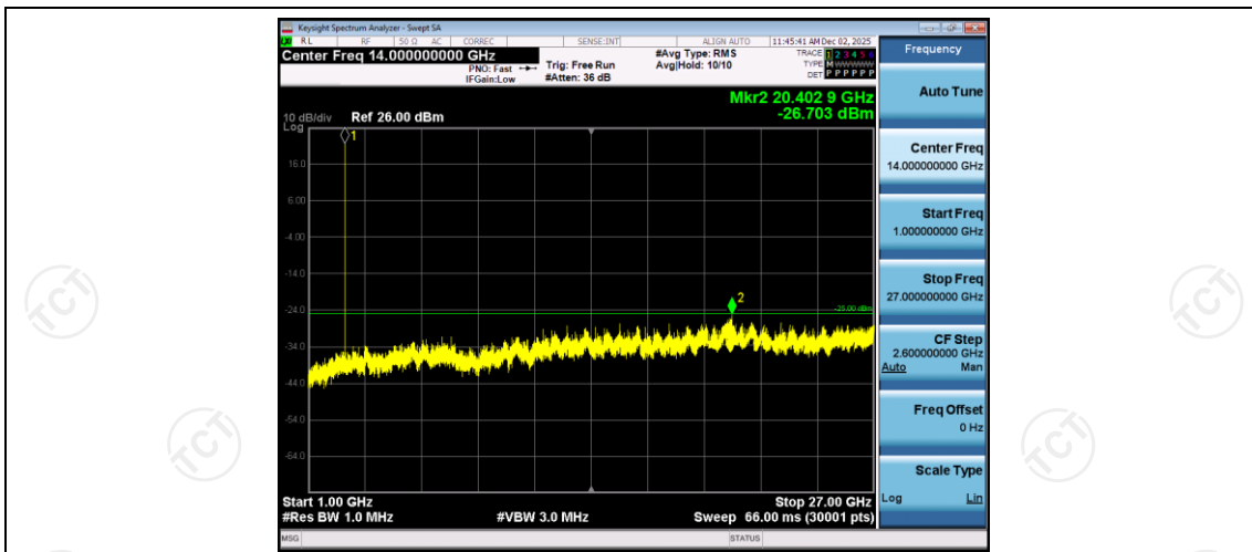
Band41-5MHz-QPSK-41565-1RB#0-Range2:1000~27000MHz
