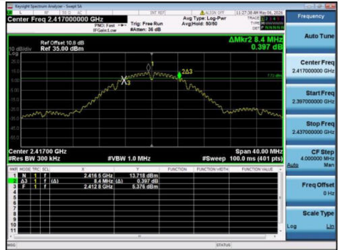
802.11b CH2
