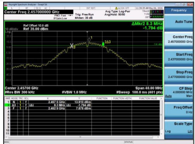
802.11b CH10
