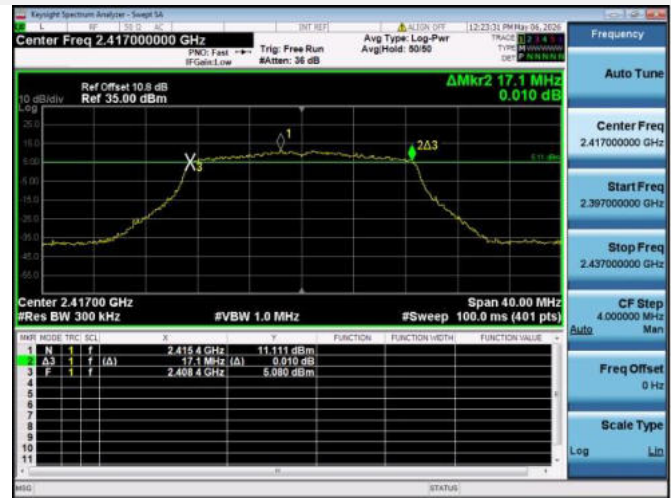
802.11n-20MHz CH2
