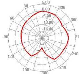
2690.000MHz E1
