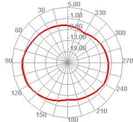
2300.000MHz H
