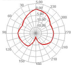
2300.000MHz E1
