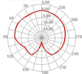
2300.000MHz E2
