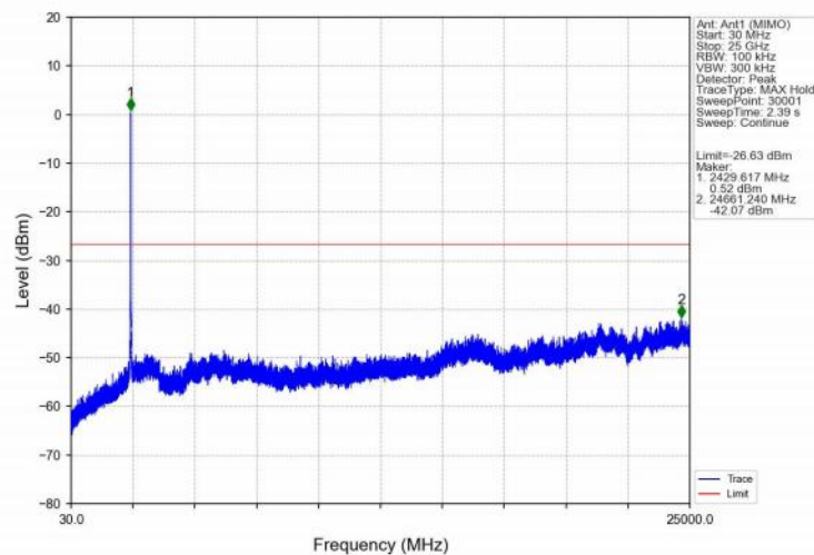
802.11ax(HEW20)_MCH_2437MHz_SU_/_Ant1 (MIMO)_NTNV
