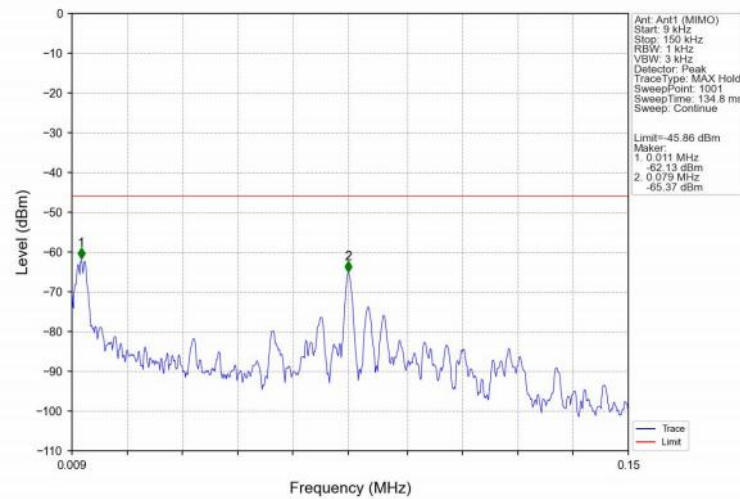
802.11n(HT20)_HCH_2462MHz_Ant1 (MIMO)_NTNV
