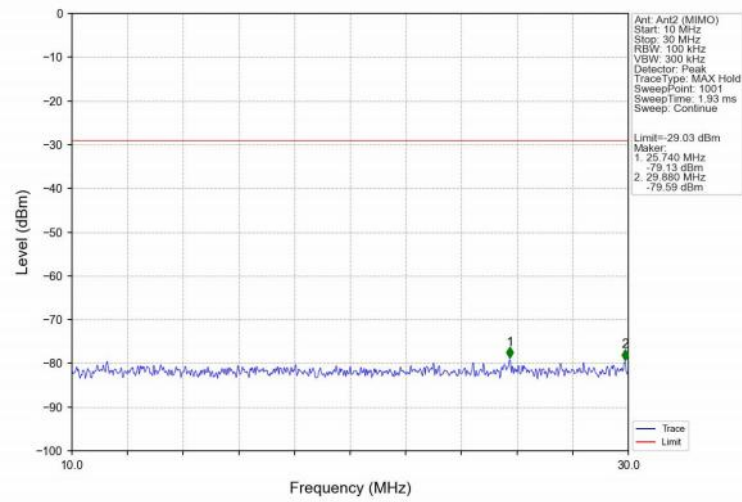
802.11n(HT40)_HCH_2452MHz_Ant2 (MIMO)_NTNV
