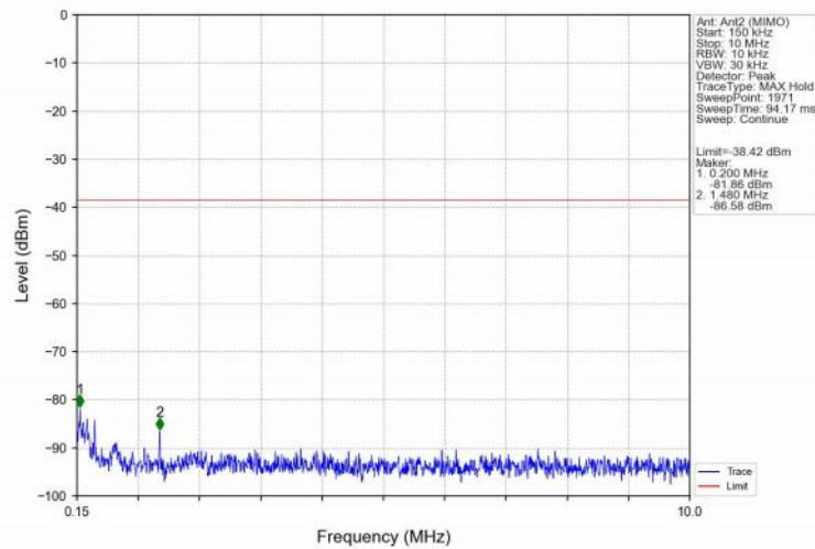
802.11n(HT40)_LCH_2422MHz_Ant2 (MIMO)_NTNV
