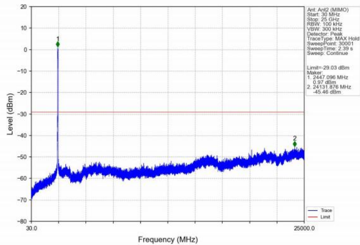
802.11n(HT40)_HCH_2452MHz_Ant2 (MIMO)_NTNV
