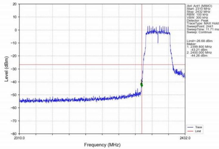
802.11n(HT20)_LCH_2412MHz_Ant1 (MIMO)_NTNV
