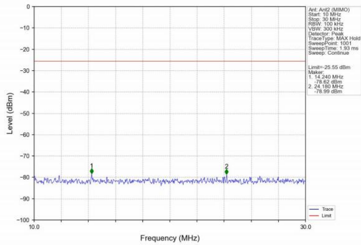
802.11n(HT20)_LCH_2412MHz_Ant2 (MIMO)_NTNV
