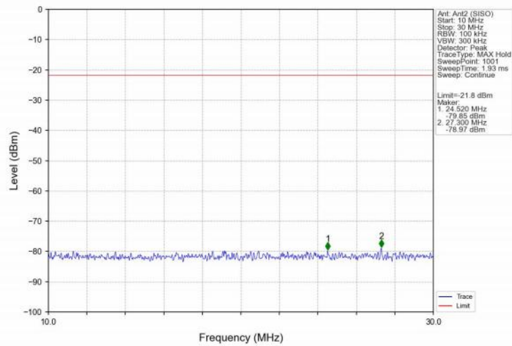
802.11b_LCH_2412MHz_Ant2 (SISO)_NTNV
