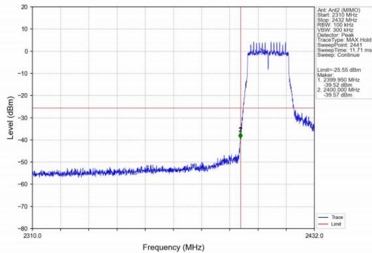
802.11n(HT20)_LCH_2412MHz_Ant2 (MIMO)_NTNV
