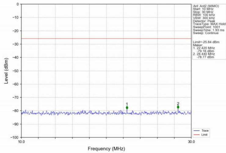
802.11n(HT20)_MCH_2437MHz_Ant2 (MIMO)_NTNV
