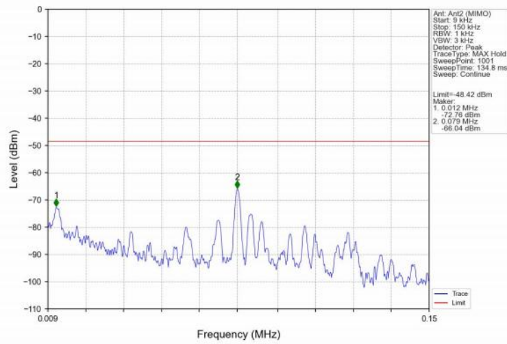
802.11n(HT40)_LCH_2422MHz_Ant2 (MIMO)_NTNV
