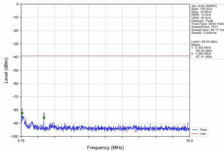
802.11n(HT40)_HCH_2452MHz_Ant2 (MIMO)_NTNV
