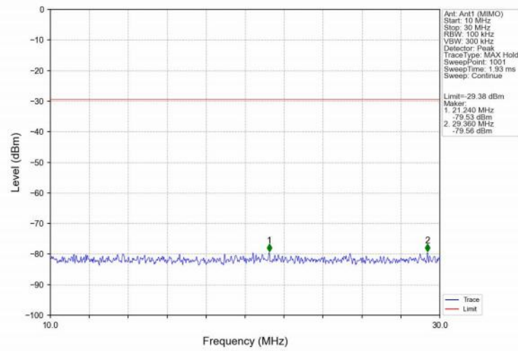
802.11n(HT40)_MCH_2437MHz_Ant1 (MIMO)_NTNV
