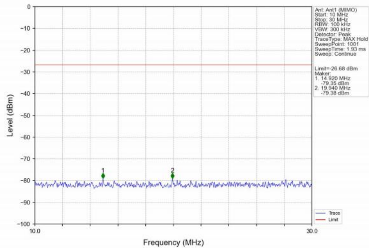
802.11n(HT20)_LCH_2412MHz_Ant1 (MIMO)_NTNV
