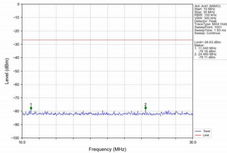
802.11ax(HEW20)_MCH_2437MHz_SU_/_Ant1 (MIMO)_NTNV
