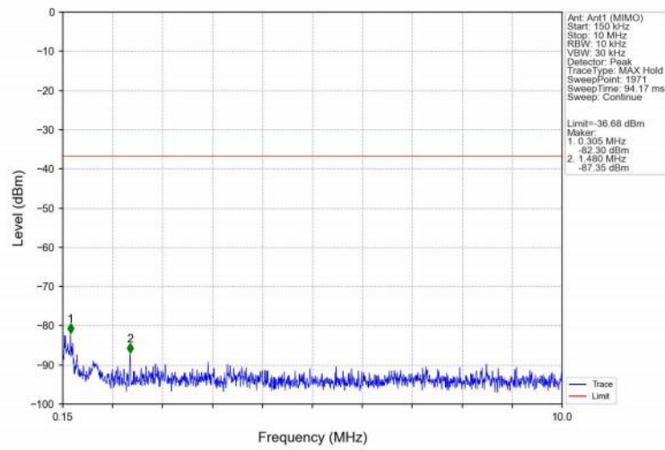
802.11n(HT20)_LCH_2412MHz_Ant1 (MIMO)_NTNV
