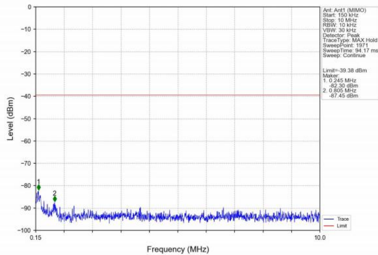
802.11n(HT40)_MCH_2437MHz_Ant1 (MIMO)_NTNV
