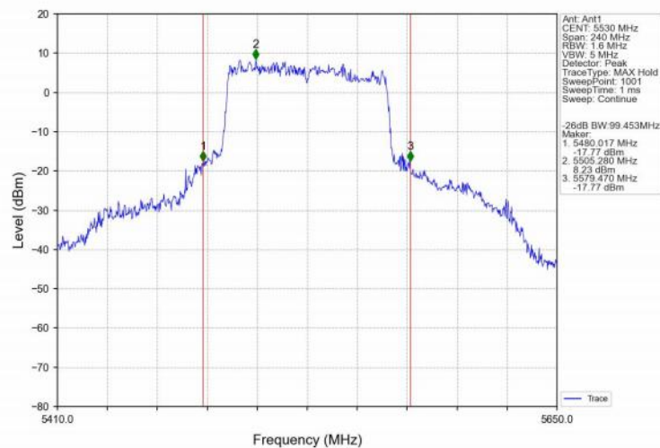
802.11ax(HEW80)_LCH_5530MHz_SU / _Ant1_NTNV
