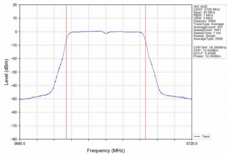
802.11n(HT20)_HCH_5700MHz_Ant2_NTNV
