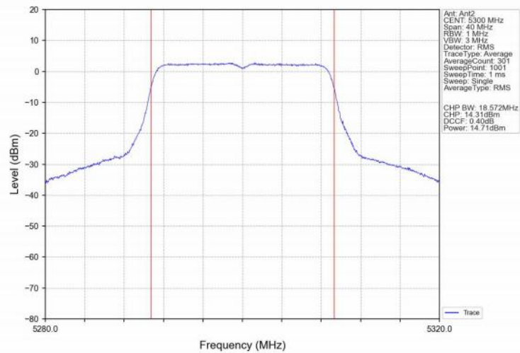
802.11n(HT20)_MCH_5300MHz_Ant2_NTNV
