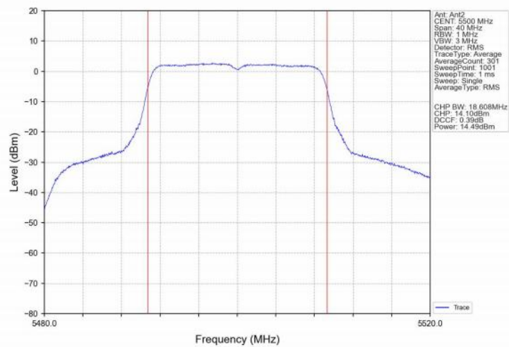
802.11n(HT20)_LCH_5500MHz_Ant2_NTNV
