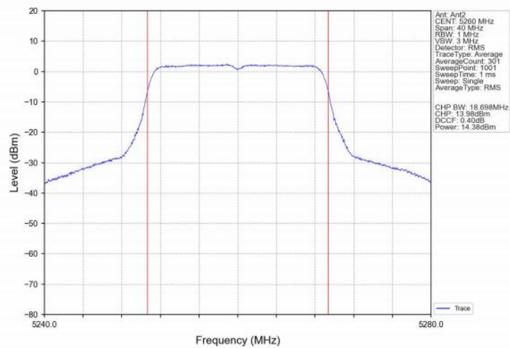
802.11n(HT20)_LCH_5260MHz_Ant2_NTNV
