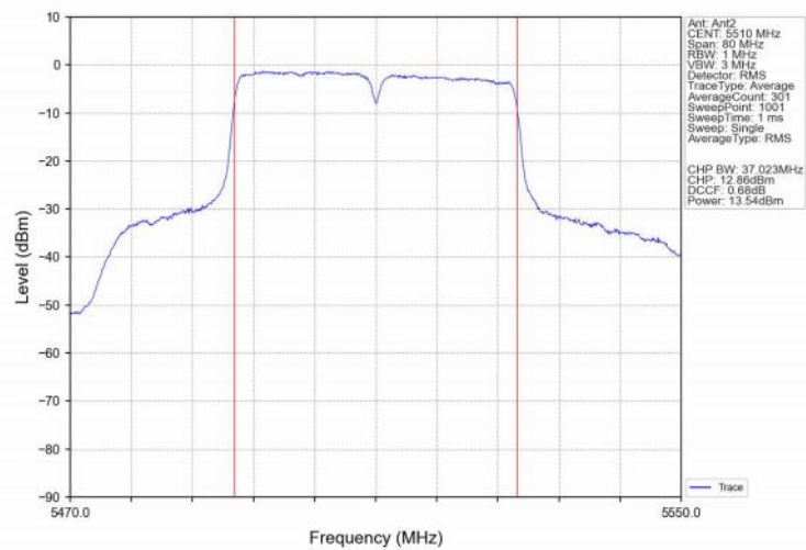
802.11n(HT40)_LCH_5510MHz_Ant2_NTNV
