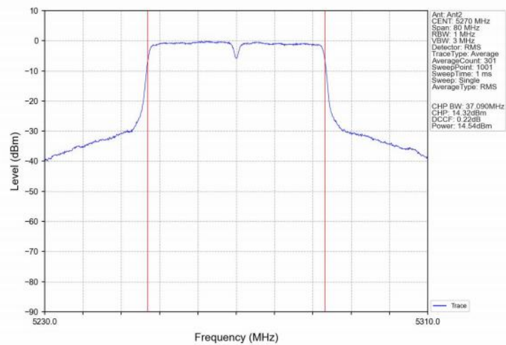
802.11ac(VHT40)_LCH_5270MHz_Ant2_NTNV
