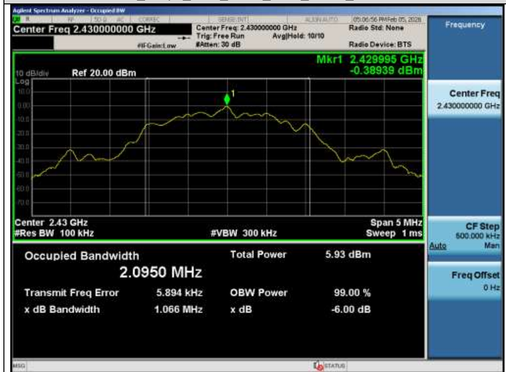
Test_Graph_2.4G_ANT1_2430_GFSK_DTSBW
