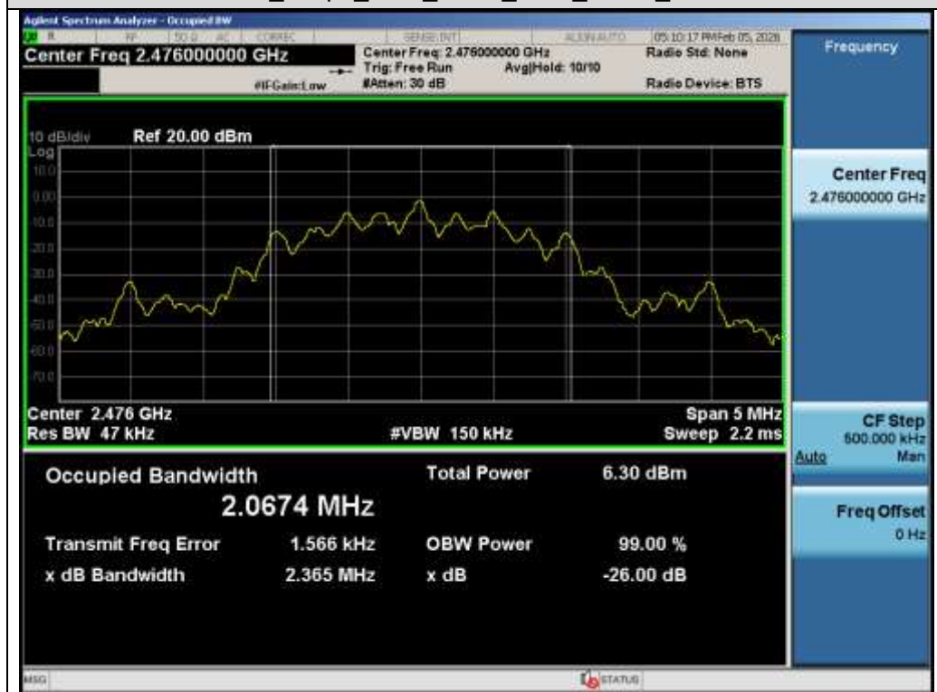
Test_Graph_2.4G_ANT1_2476_GFSK_OBW
