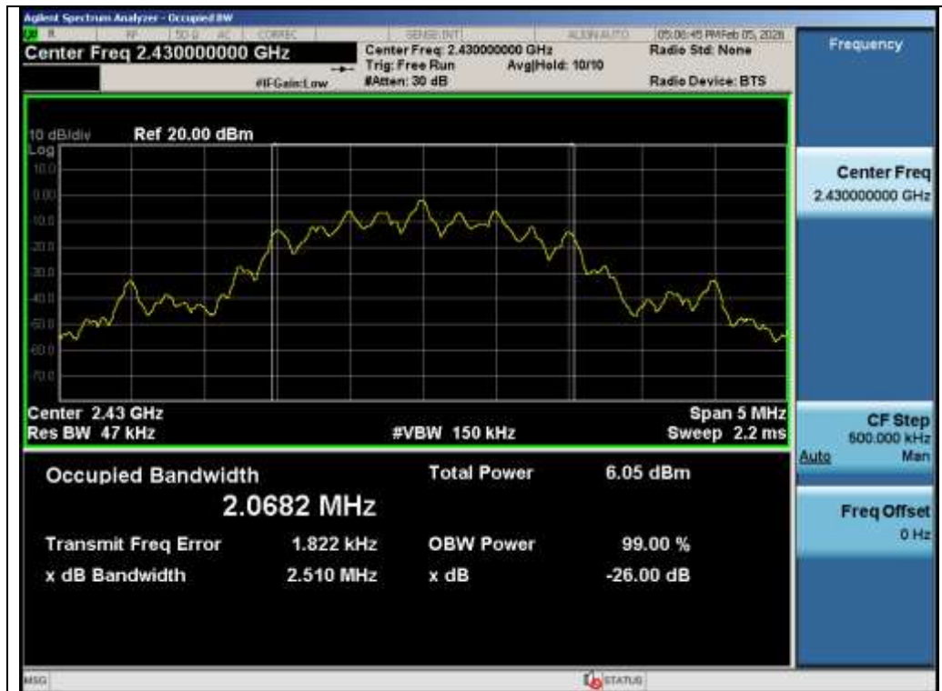
Test_Graph_2.4G_ANT1_2430_GFSK_OBW
