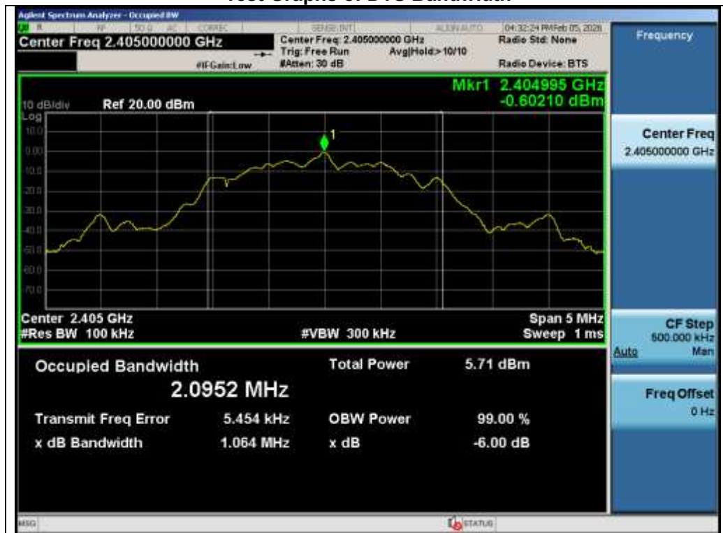
Test_Graph_2.4G_ANT1_2405_GFSK_DTSBW
