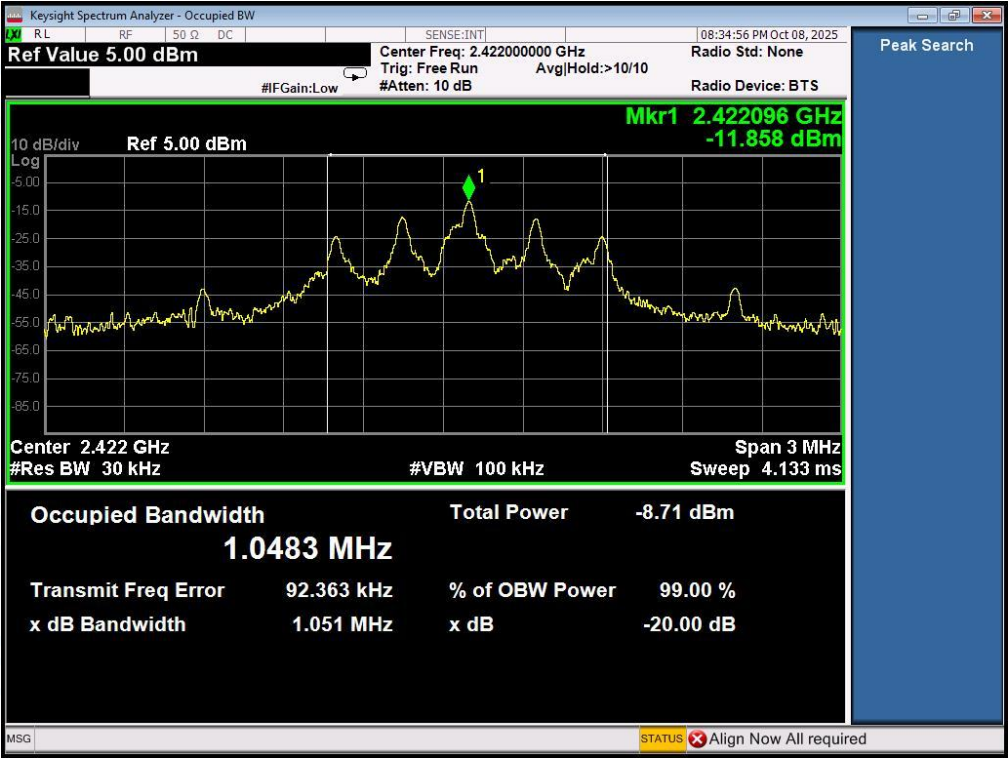
2422MHz
