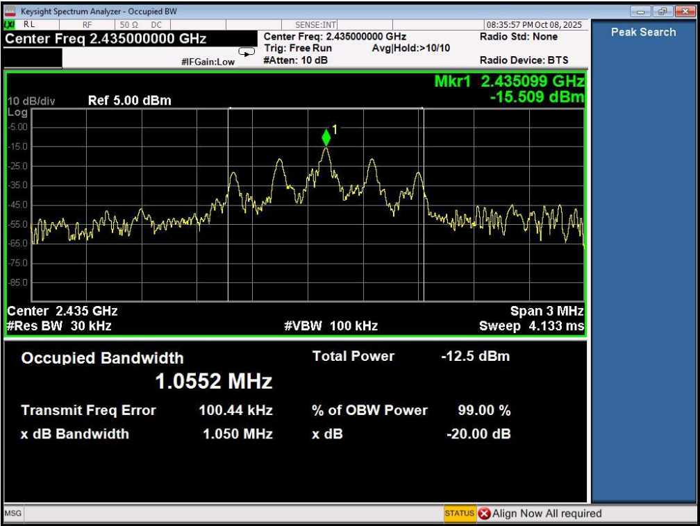
2435MHz
