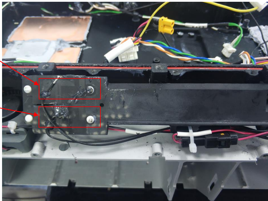
Wi Fi chain 1 Antenna
