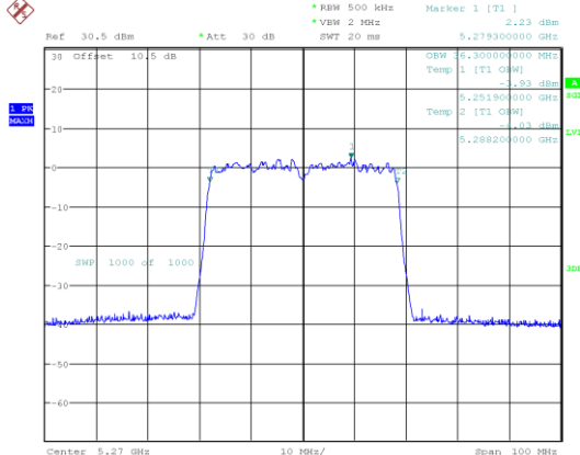
802.11ac40_5270MHz
