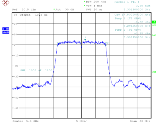
802.11ac20_5300MHz
