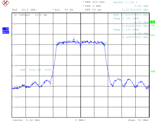
802.11ac20_5320MHz
