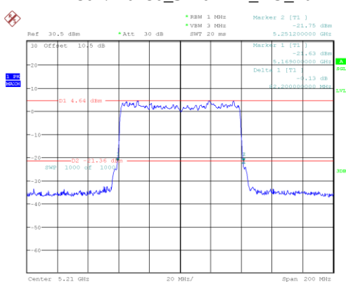
802.11ax80_5210MHz_RU_Full
