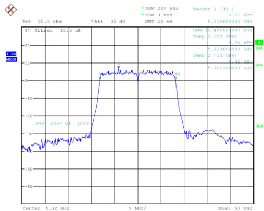
802.11a_5320MHz
