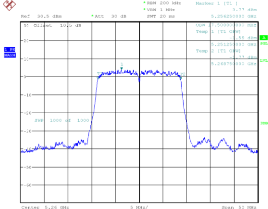
802.11ac20_5260MHz
