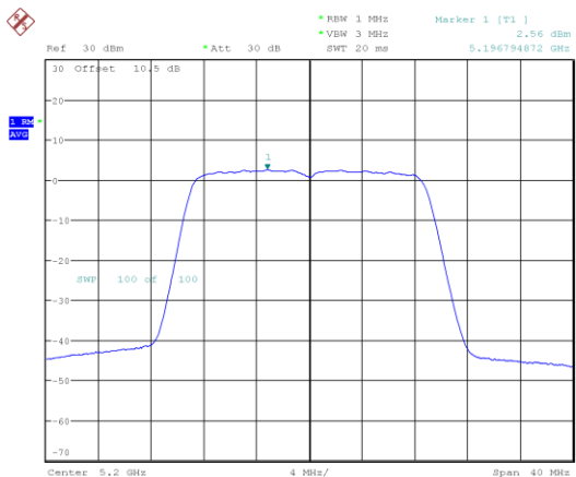
802.11ac20_5200MHz
