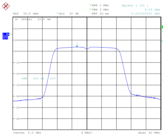
802.11ac20_5300MHz
