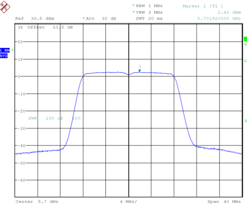
802.11a_5700MHz
