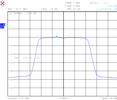
802.11ac20_5500MHz
