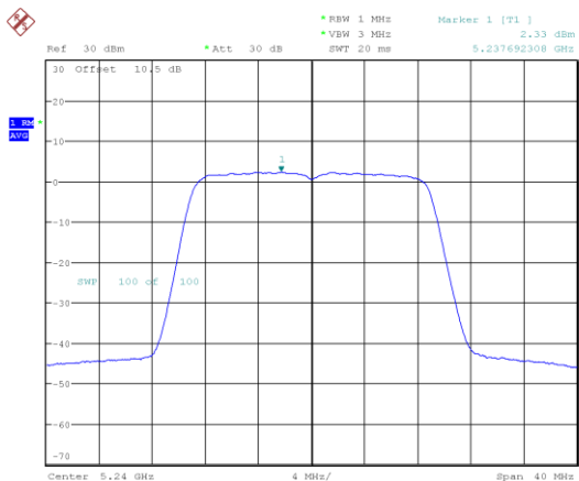
802.11ac20_5240MHz
