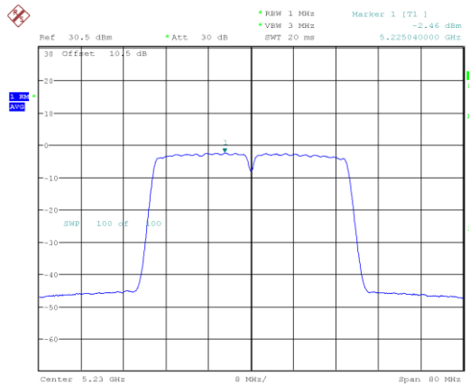
802.11ac40_5230MHz
