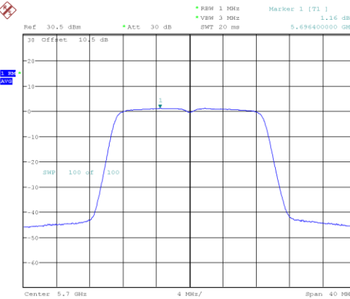
802.11ac20_5700MHz
