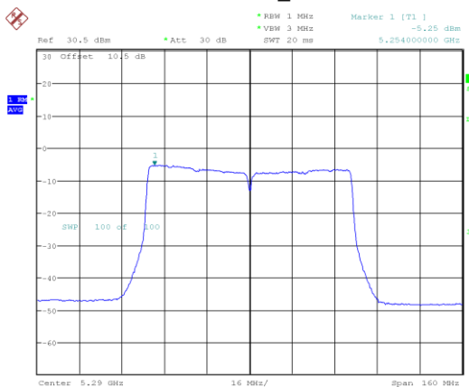
802.11ac80_5290MHz
