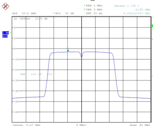
802.11ac40_5270MHz
