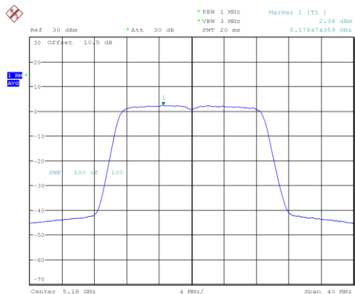
802.11ac20_5180MHz
