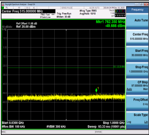
2.4GHz-Ant1-2402-30~1000-PASS
