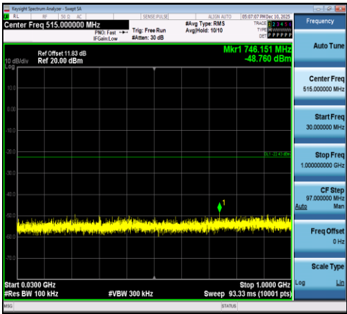
2.4GHz-Ant1-2440-30~1000-PASS
