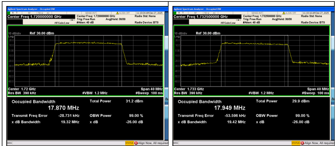
Band4-20MHz-QPSK-20050-100RB#0-PASS
