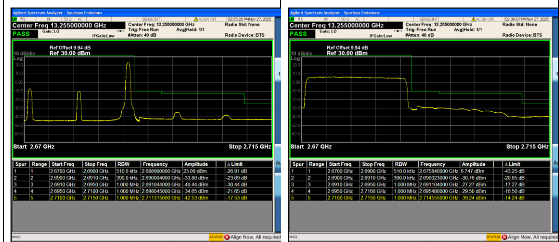
Band41_20MHz_QPSK_41490_1RB#99
