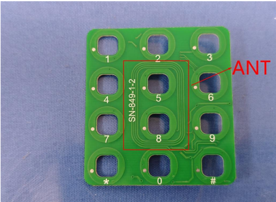
NFC ANT
