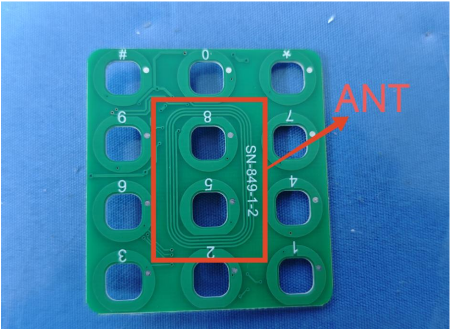
NFC ANT
