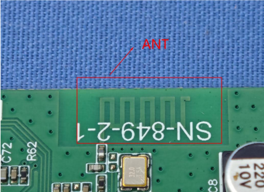
BLE ANT
