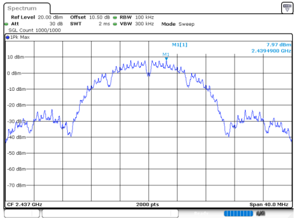
802.11b_2437MHz
