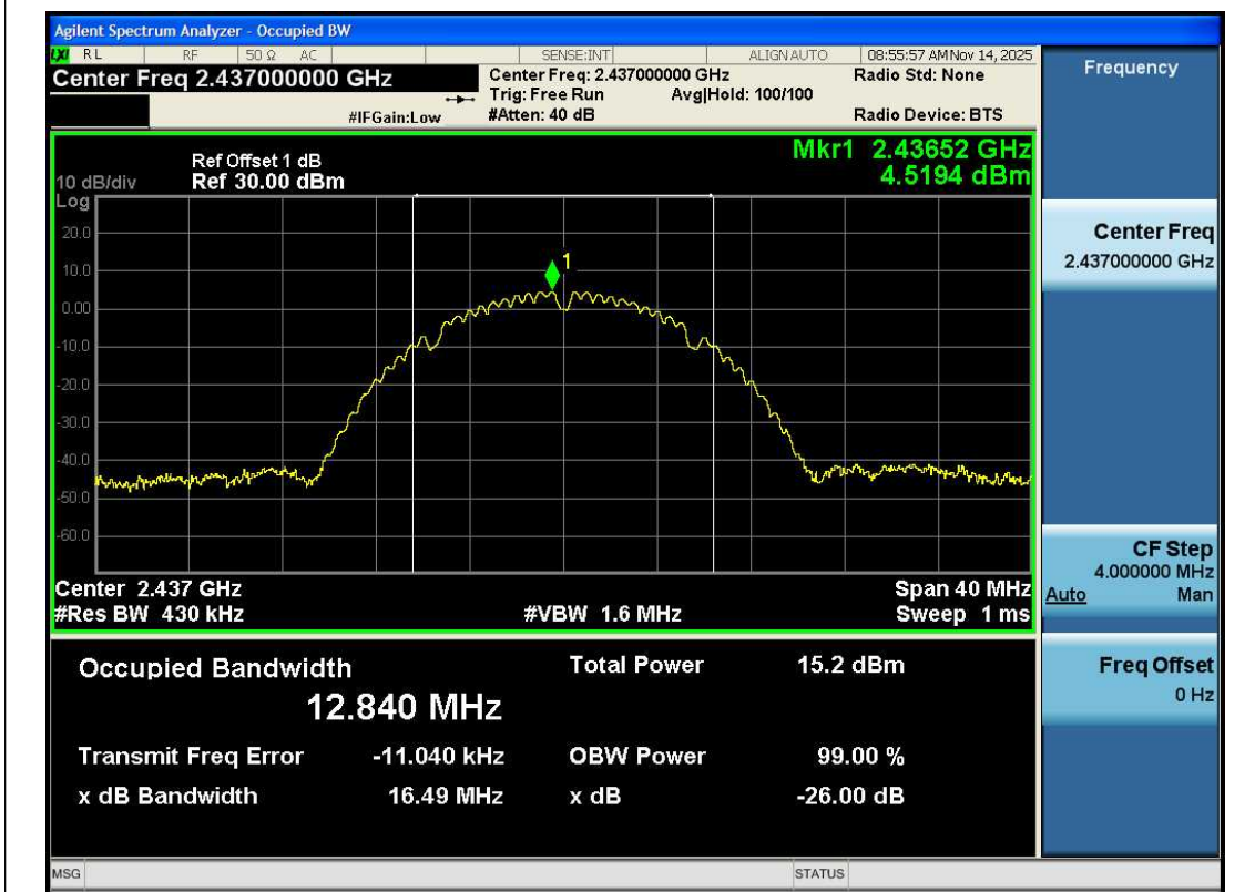
11B-Ant1-2437
