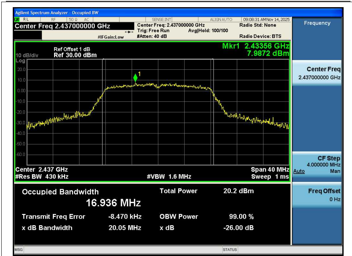
11G-Ant1-2437
