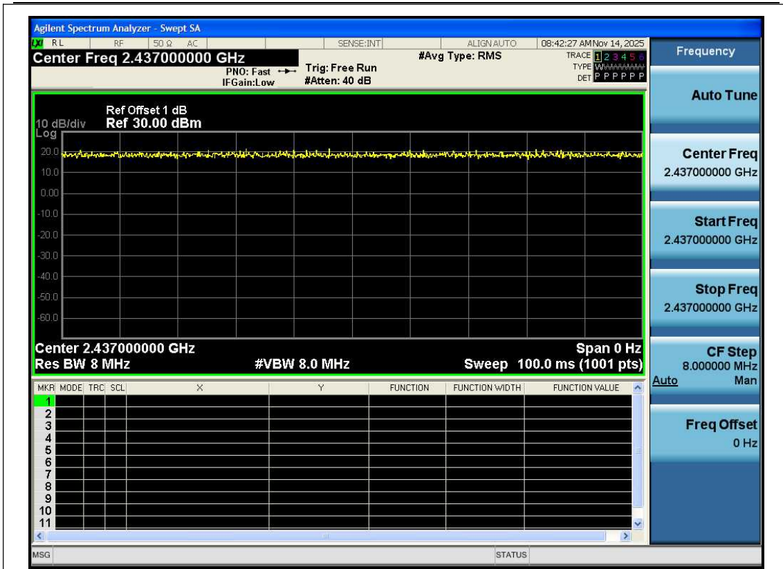
NTNV-11G-Ant1-2437
