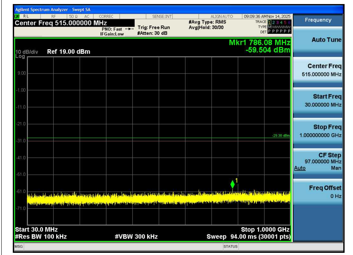
11G-Ant1-2437-30~1000-PASS
