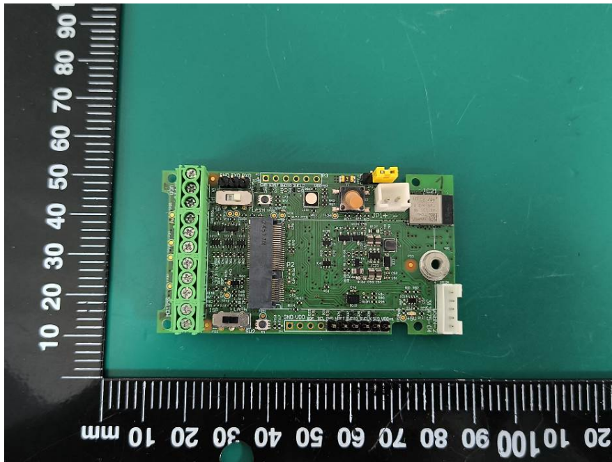
BT Module
