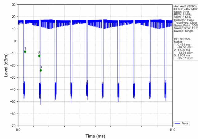
802.11b_HCH_2462MHz_Ant1 (SISO)_NTNV
