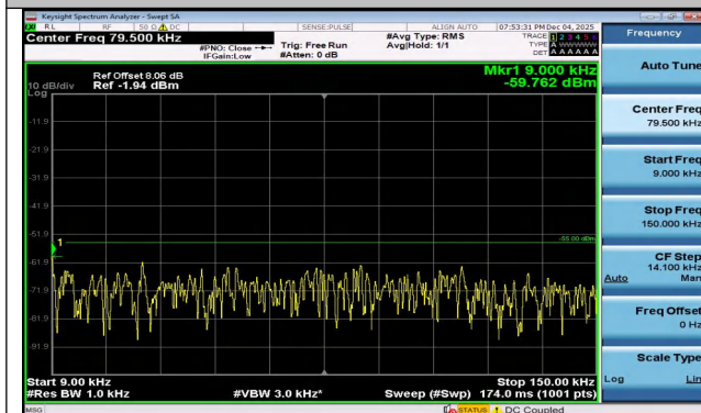
Band7-10MHz-QPSK-20800-50RB#0-0.009~0.15-PASS
