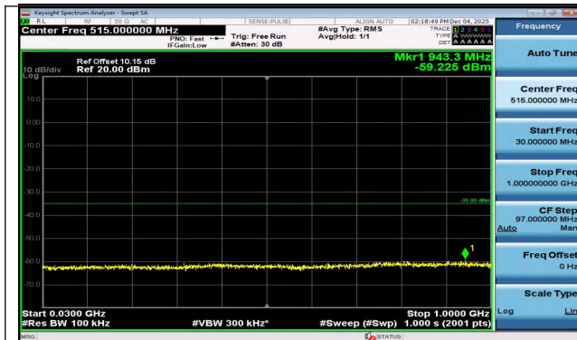
Band7-10MHz-QPSK-20800-50RB#0-30~1000-PASS
