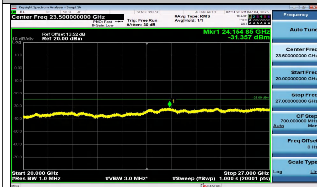
Band7-15MHz-16QAM-20825-1RB#74-20000~27000-PASS
