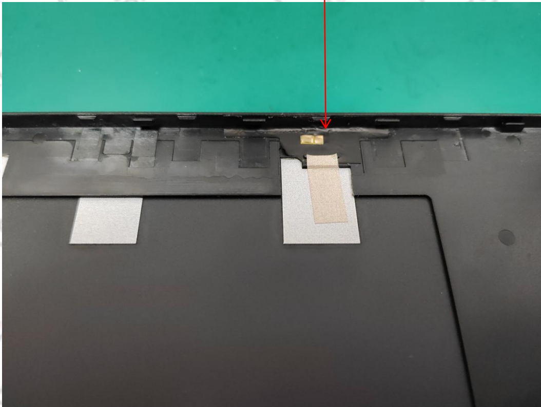
BT&WiFi 2.4/5G_ANT
