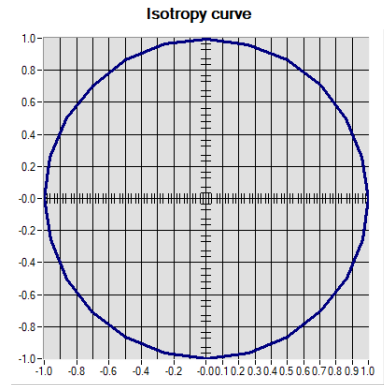
Isotropy: +/-0.25% (+/-0.01dB)
