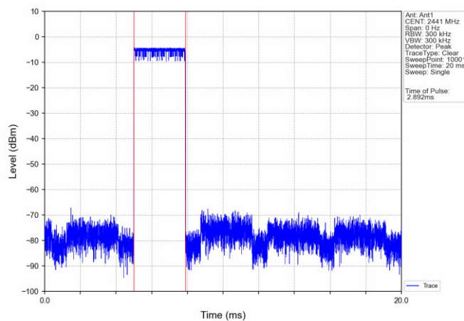
GFSK_DH5_HOPP_Ant1_NTNV
