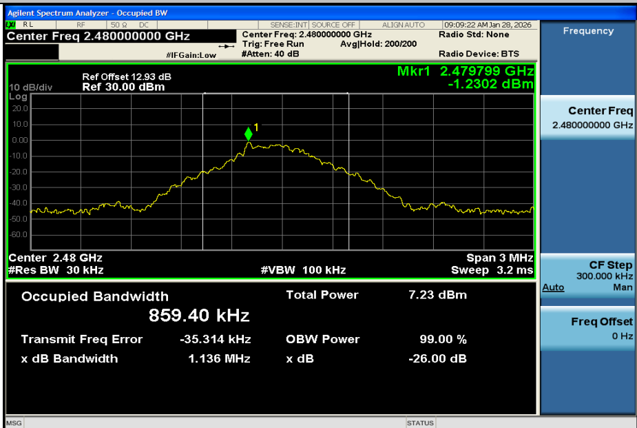
DH5-Ant1-2480
