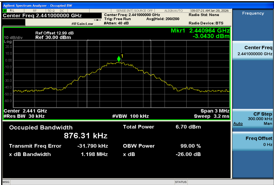
DH5-Ant1-2441
