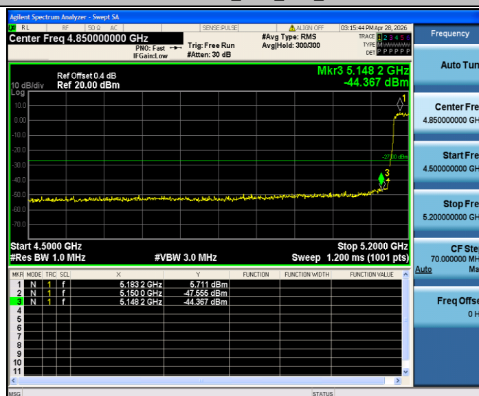
11AX40SISO_Ant2_Low_5190
